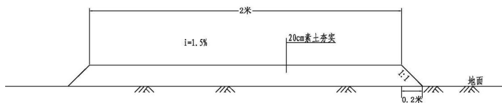
图 11-2 生产路路面结构设计图
