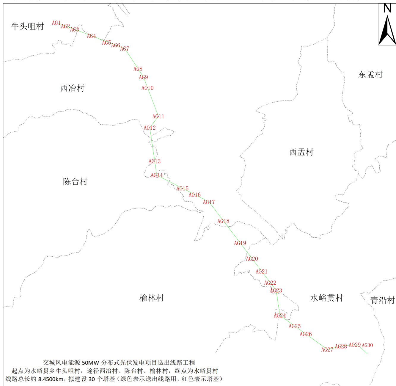
交城风电能源50MW分布式光伏发电项目送出线路工程拟选址方案图
