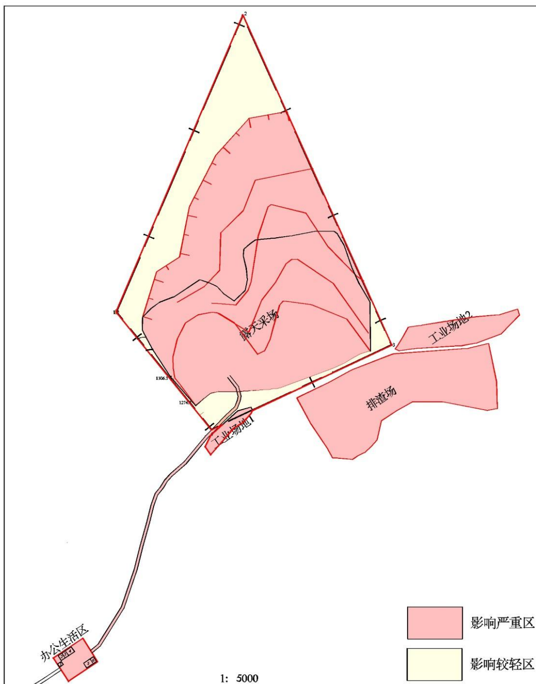
图 8-3 矿山开采对地形地貌影响现状评估分区图
