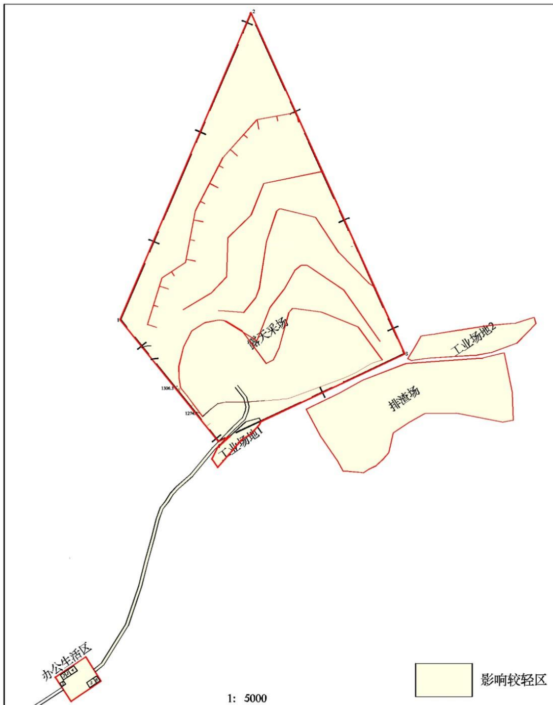
图 8-2 矿山开采对含水层影响现状评估分区图
