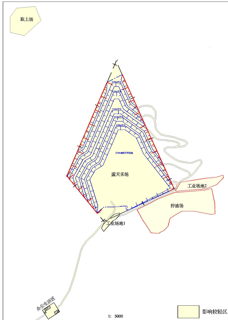
图 8-6 矿山开采对含水层影响预测评估分区图
