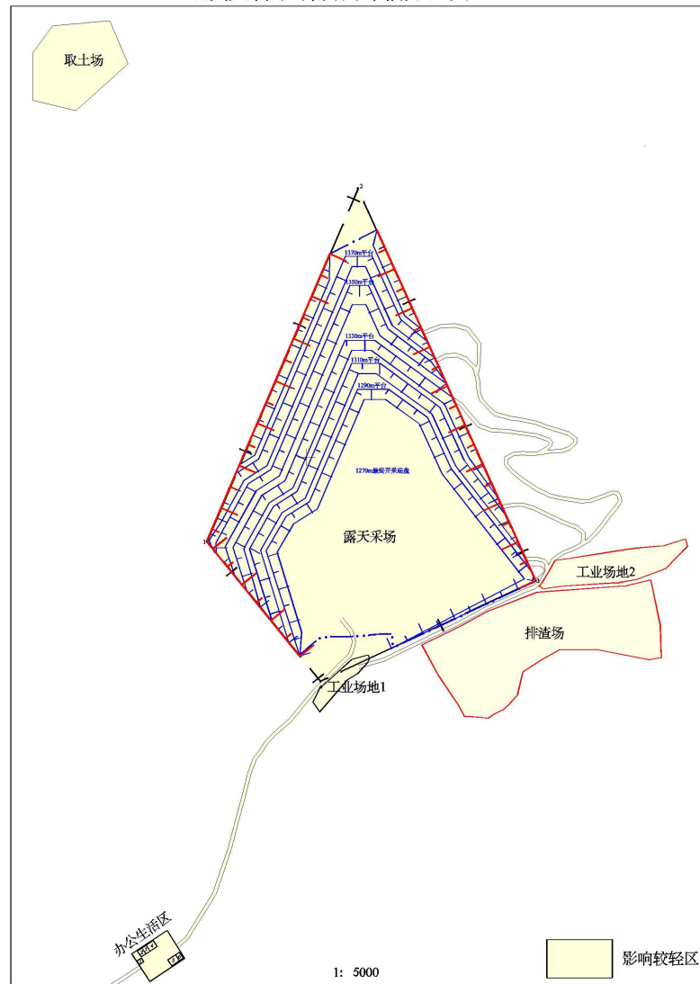
图 8-5 地质灾害影响预测评估分区图
