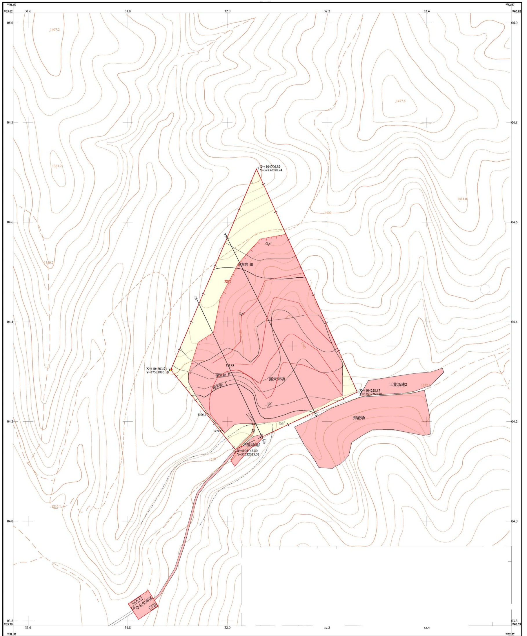
图 8-4 矿山地质环境影响现状评估图
