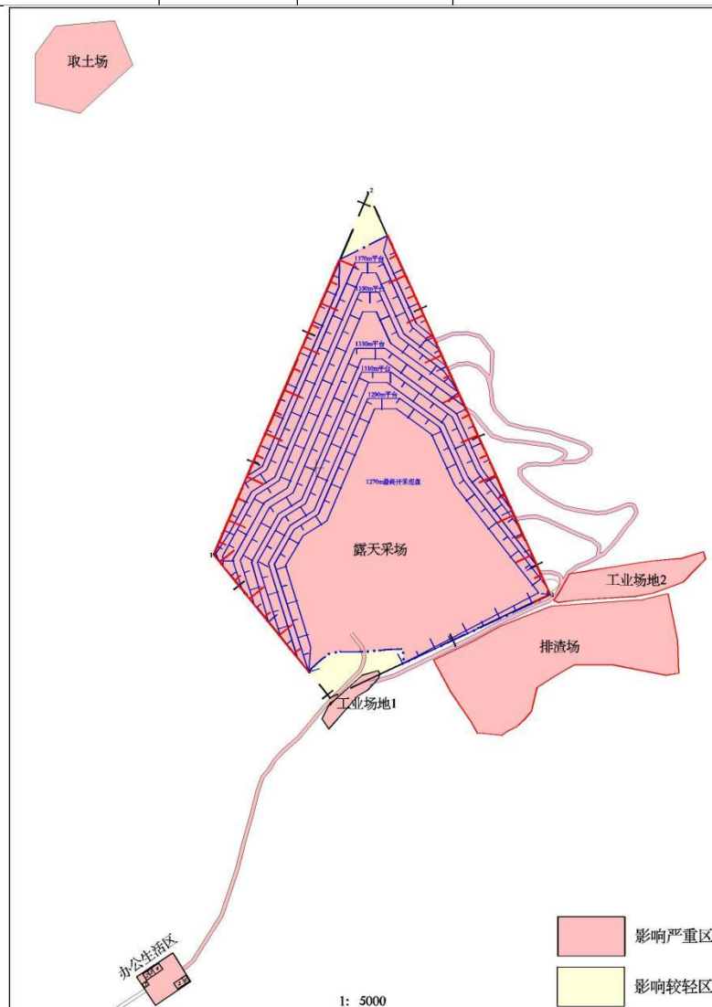
图 8-7 矿山开采对地形地貌影响预测评估分区图
