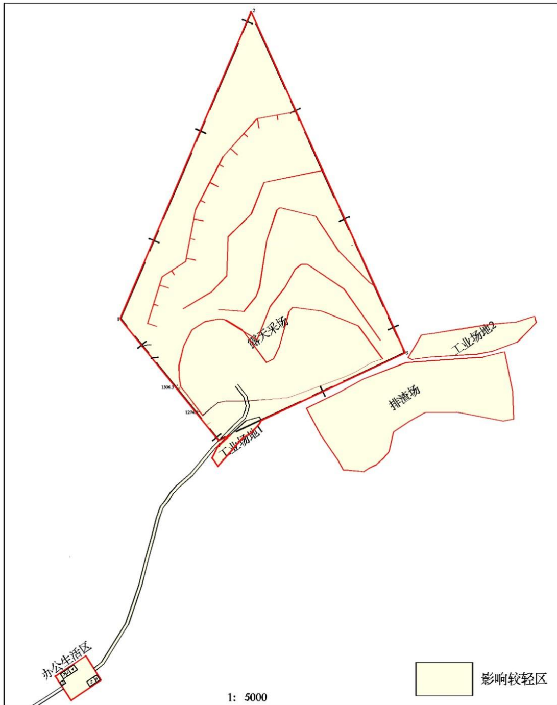
图 8-1 地质灾害影响程度现状评估分区图
