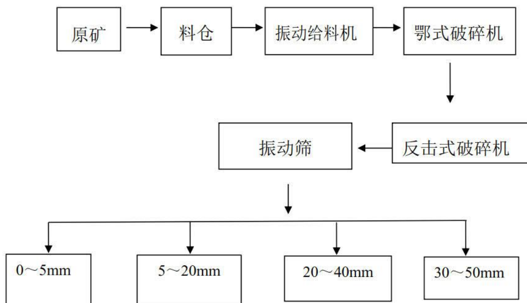
图 6-1-1 机械破碎加工工艺流程图
