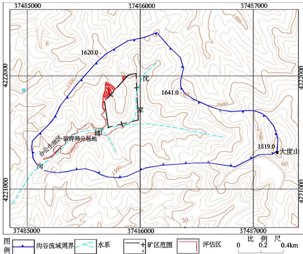
图 8-1 沟谷流域图
