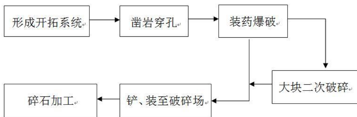
图 5-1 开采工艺图
