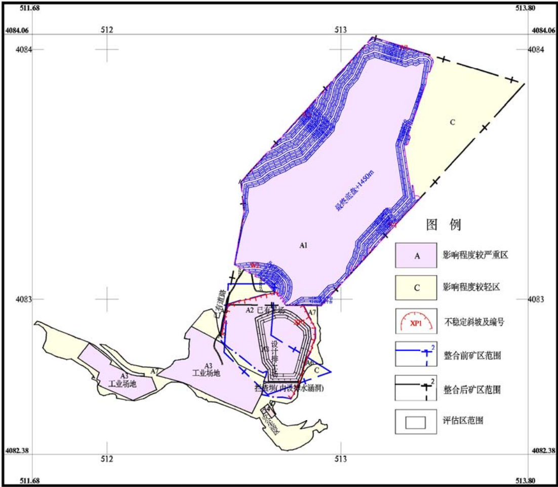
图 8-8 地质灾害预测评估分区图
