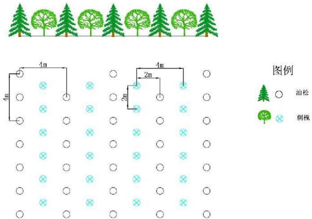
图 11-3 乔木林地造林典型设计图
