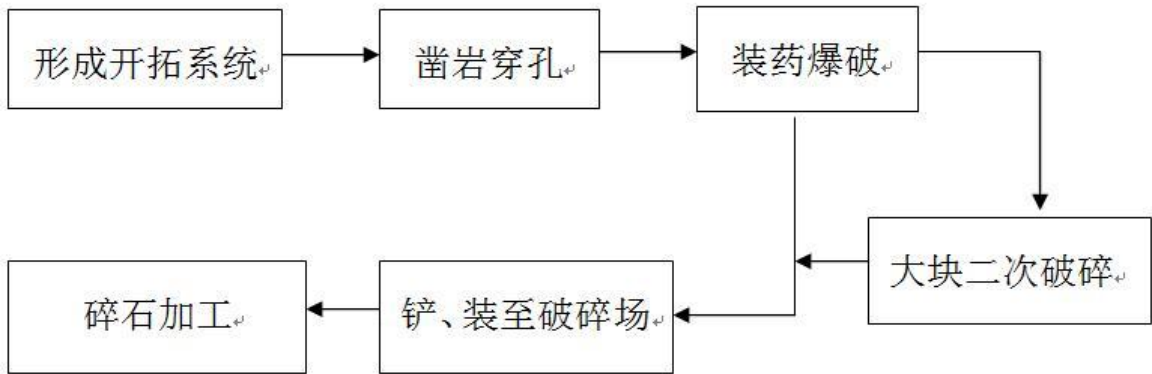
图 5-1 开采工艺图
