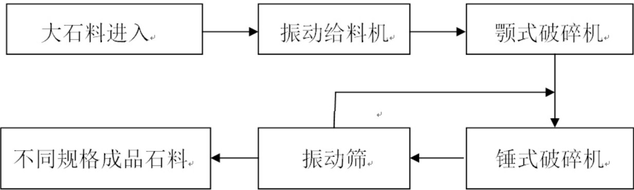
图 5-2 生产线流程图
