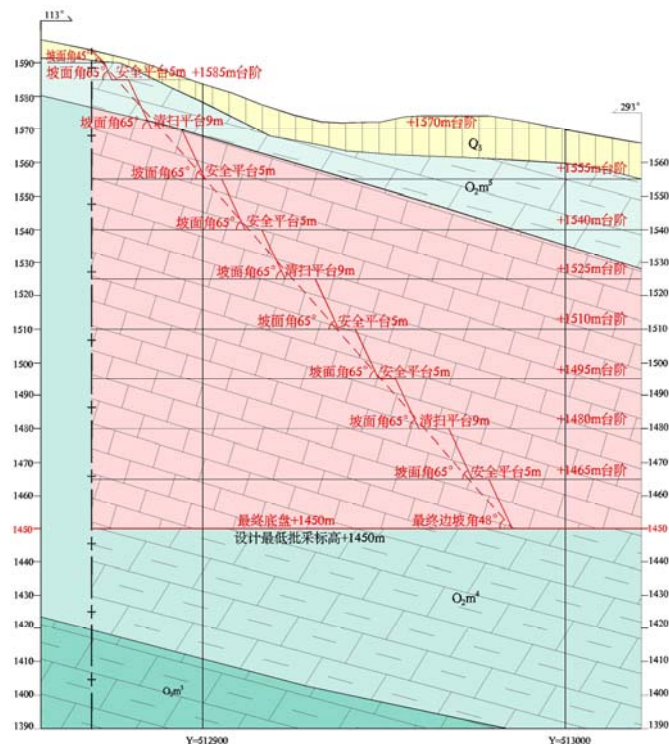
图 8-5 设计采场 W1 西部边坡地质剖面图
