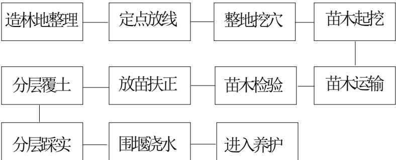
图 11-1 绿化种植施工流程示意图
