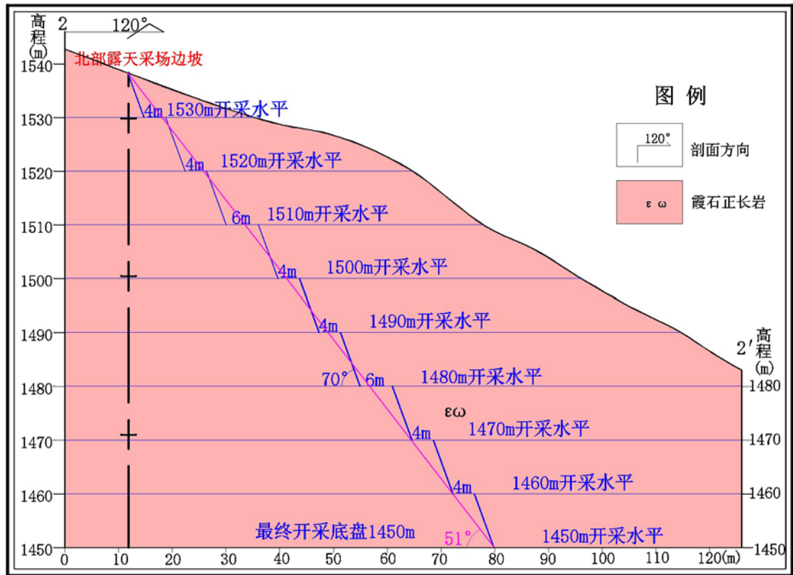
图 8-5 北部露天采场终了边坡
