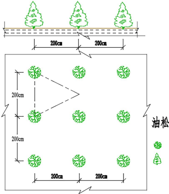
图 11-1-1 油松配置设计图
