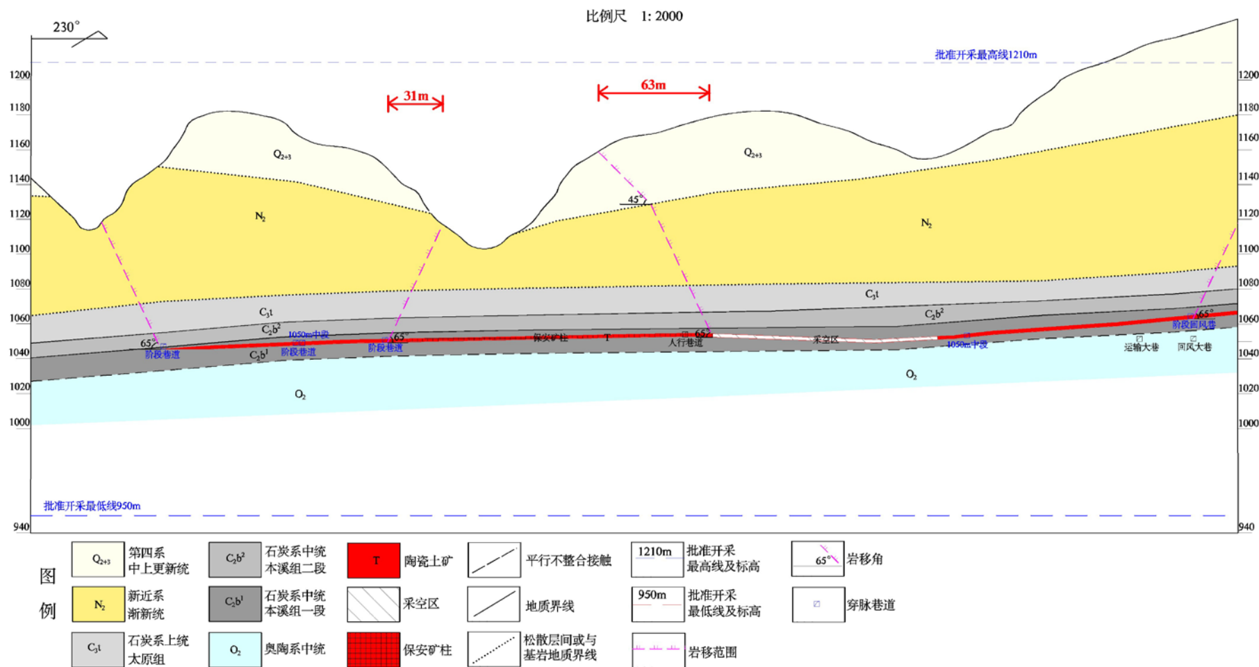
图 8-3-1 1-1' 预测陶土三矿矿层开采引发地面变形范围计算示意图
