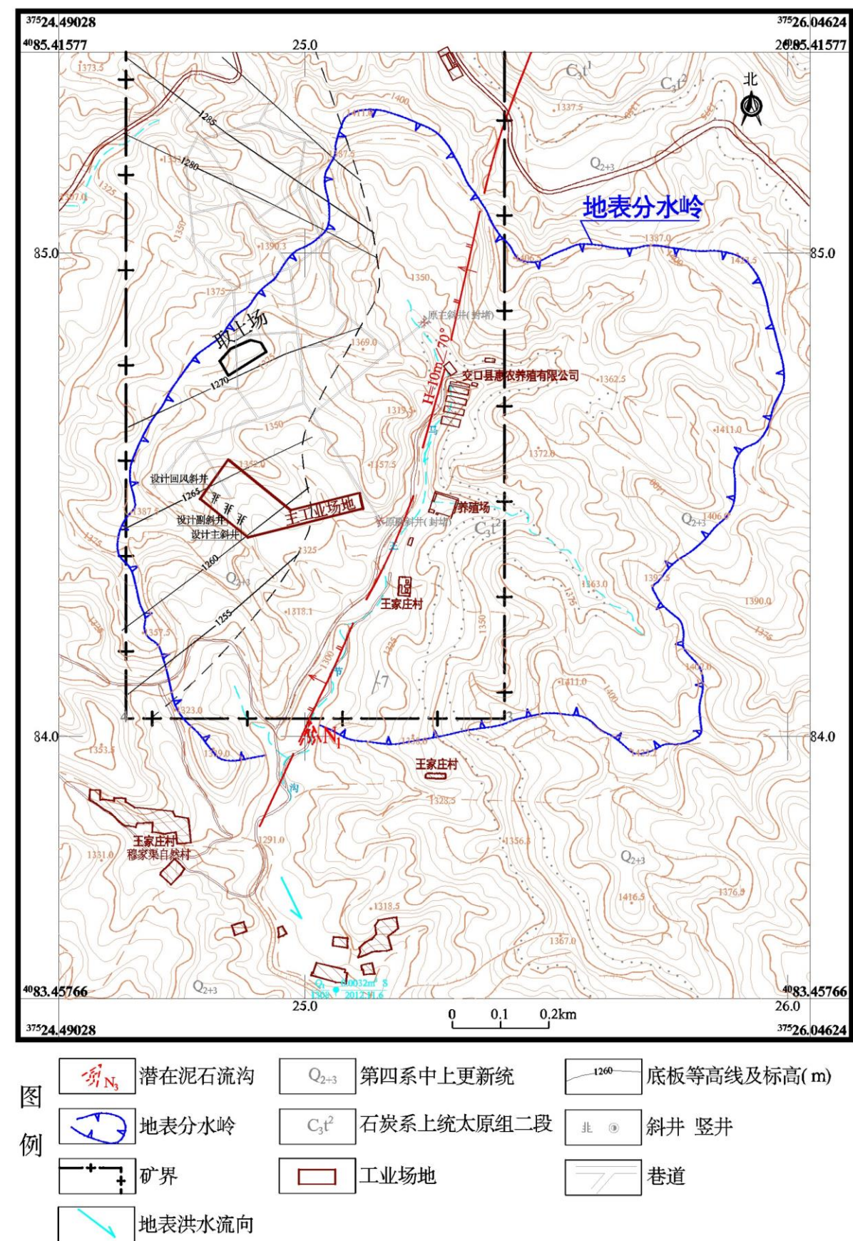
图 8-3-3 马王节沟 N 1 潜在泥石流沟示意图
