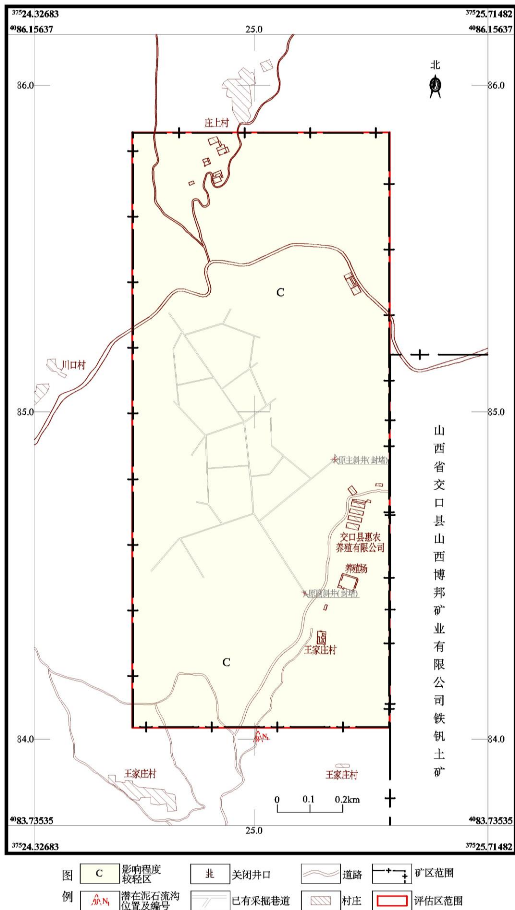
图 8-2-2 含水层影响或破坏程度现状评估分区图
