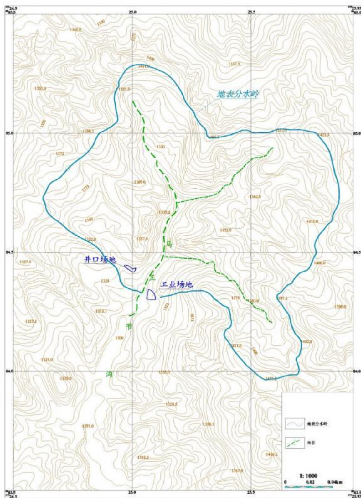
图 2-1-1 区域水系图
