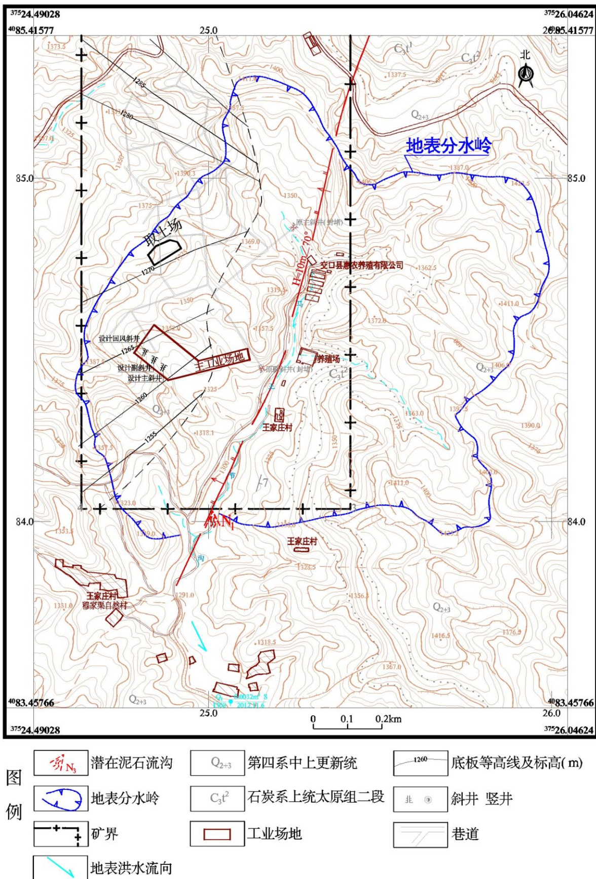
图 8-3-3 马王节沟 N 1 潜在泥石流沟示意图
