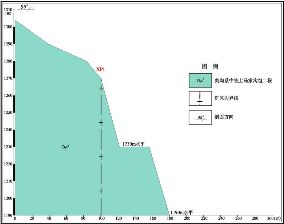
图 8-4 旧采场 XP1 边坡
