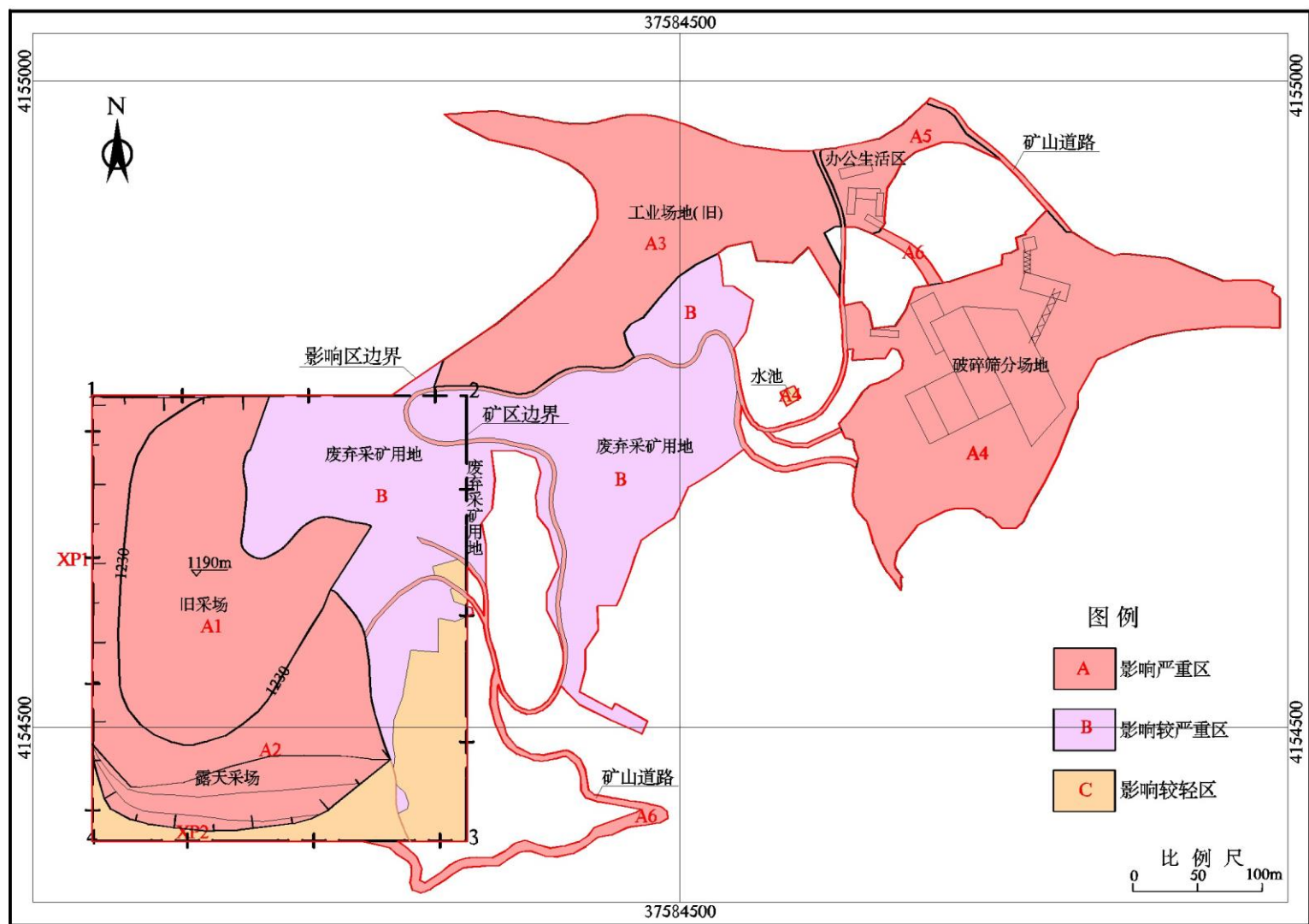
图 8-3 地形地貌影响和破坏程度现状评估分区图
