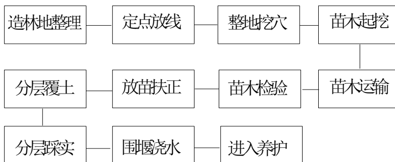
图 11-1 绿化种植施工流程图
