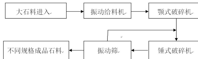
生产线流程图
