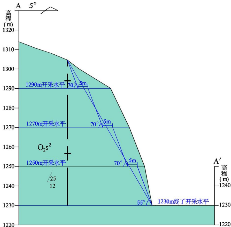
图 8-5 露天采场 XP2 边坡
