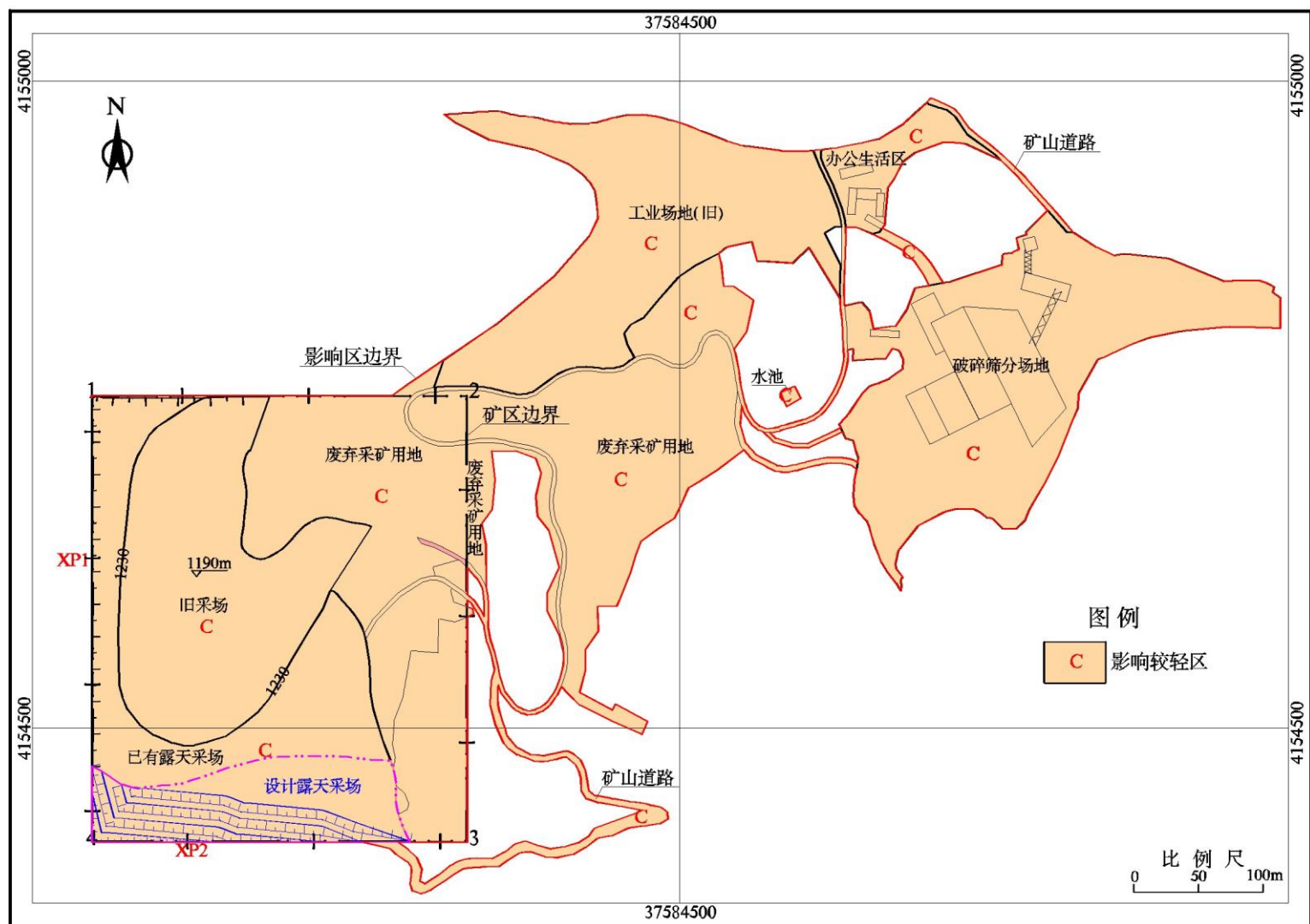
图 8-7 适用期含水层影响和破坏程度预测评估分区图
