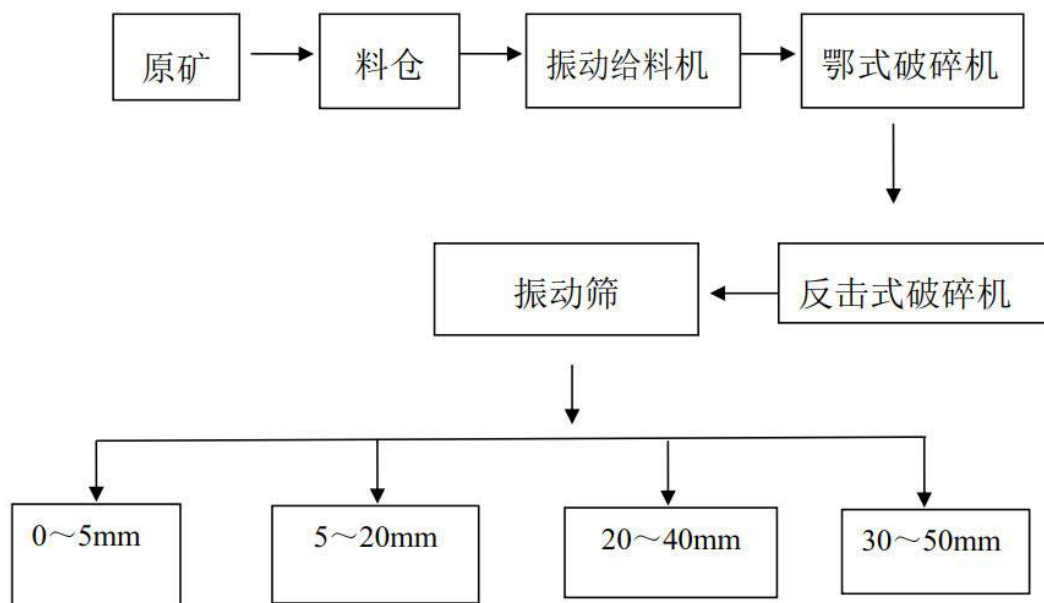
图 6-1-1 工艺流程图
