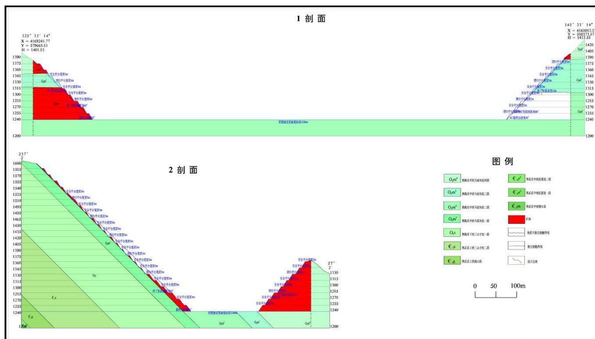
图 8-3-3 设计露天采场终了边坡剖面图
