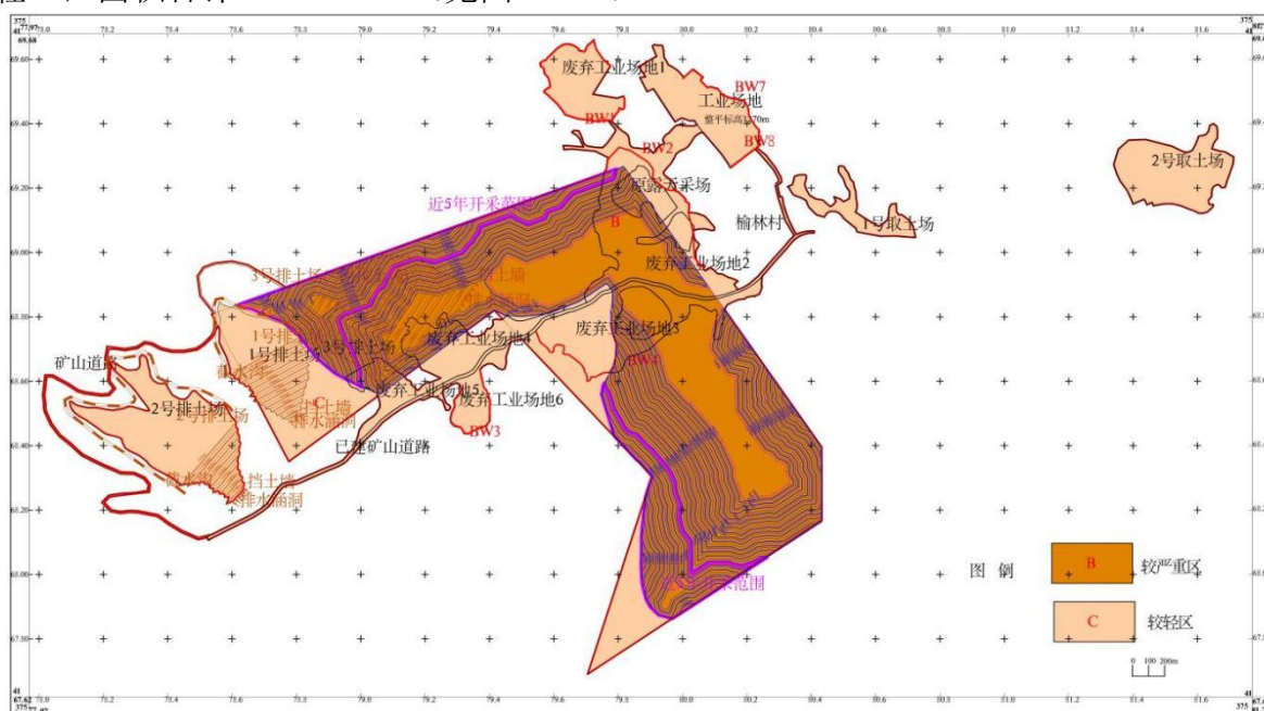
图 8-3-3 含水层影响预测评估图
