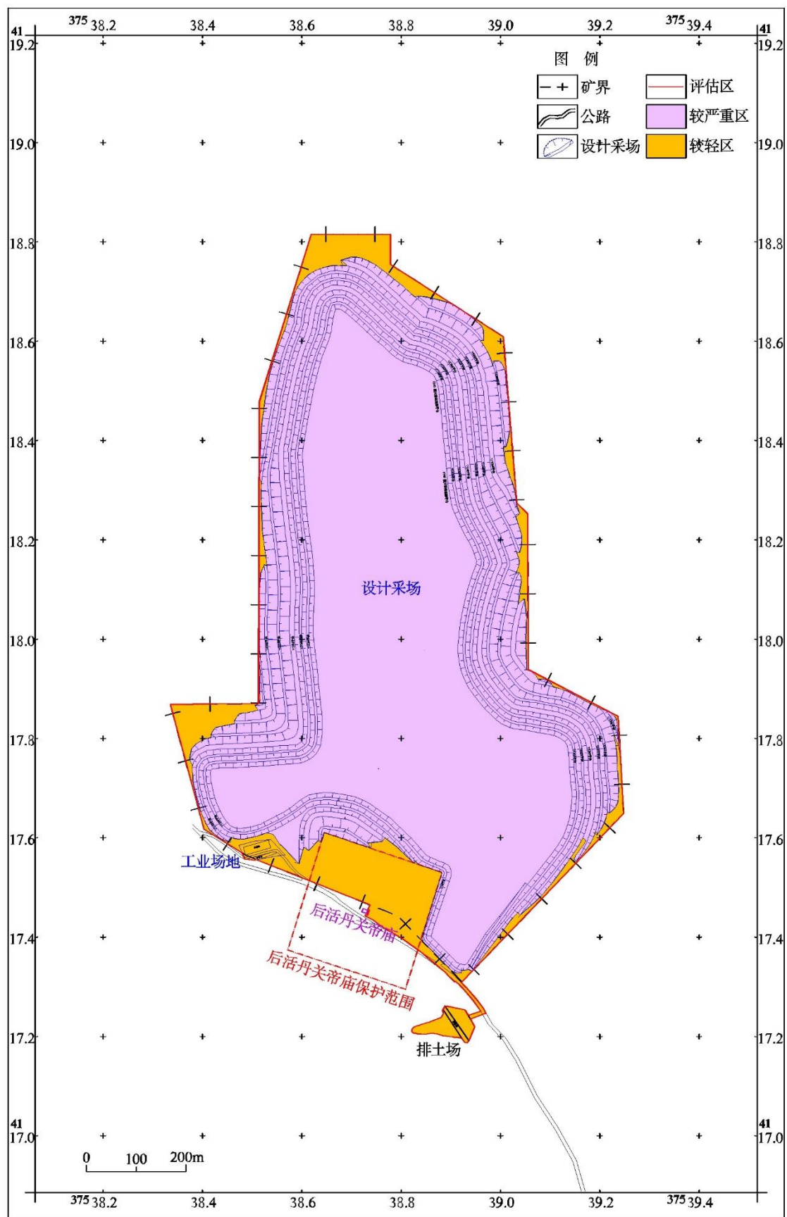
图 8-7 地质灾害危险性预测评估图
