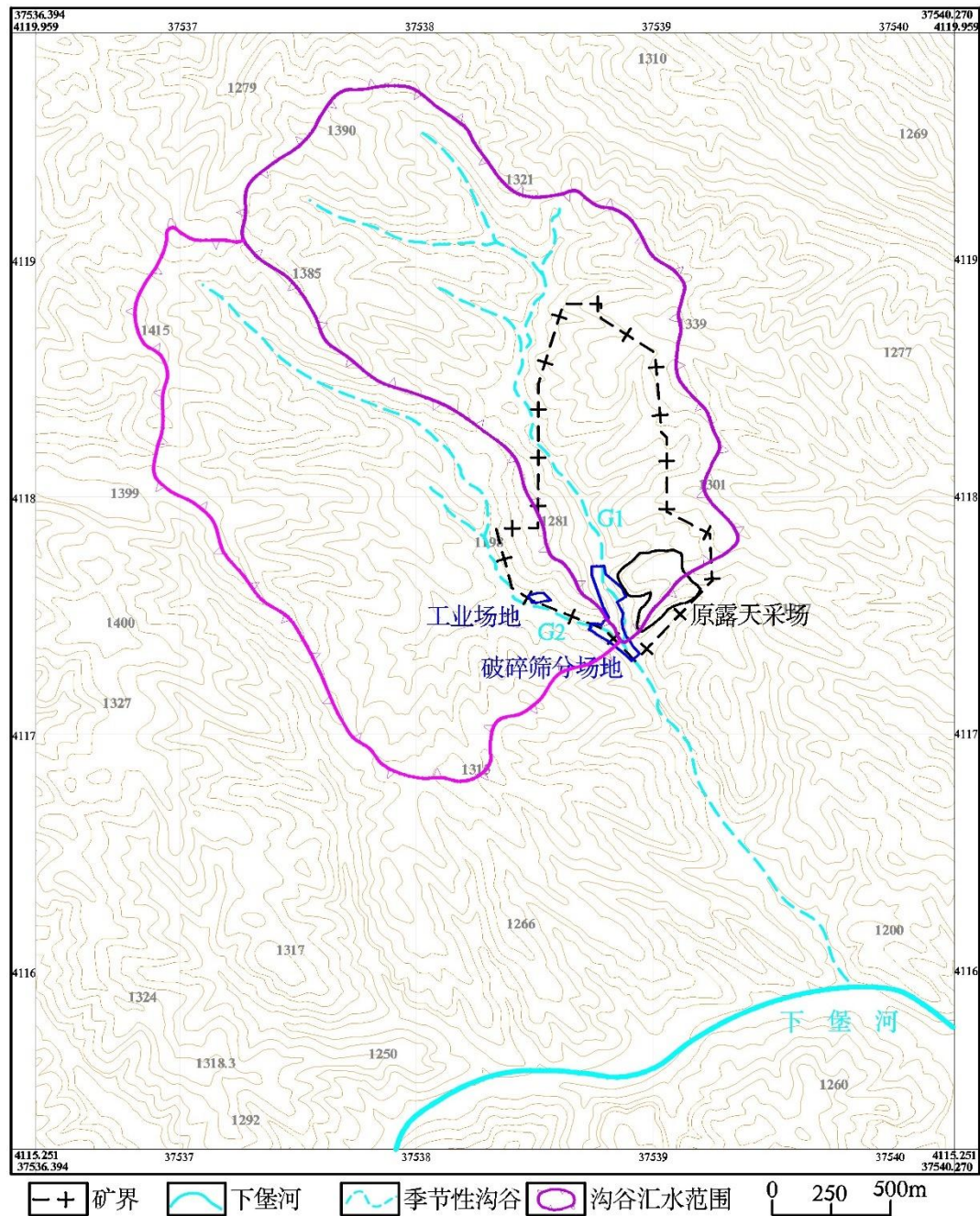
图 8-1 矿区沟谷汇水范围图
