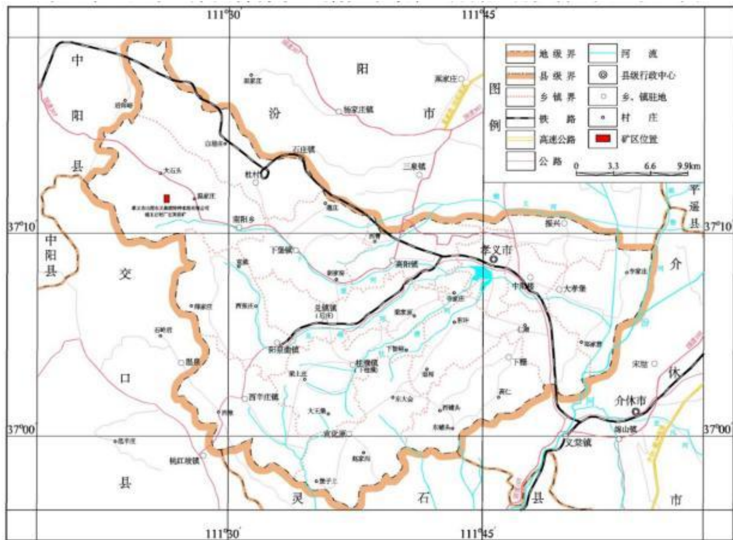
图 2-2 区域水系图
