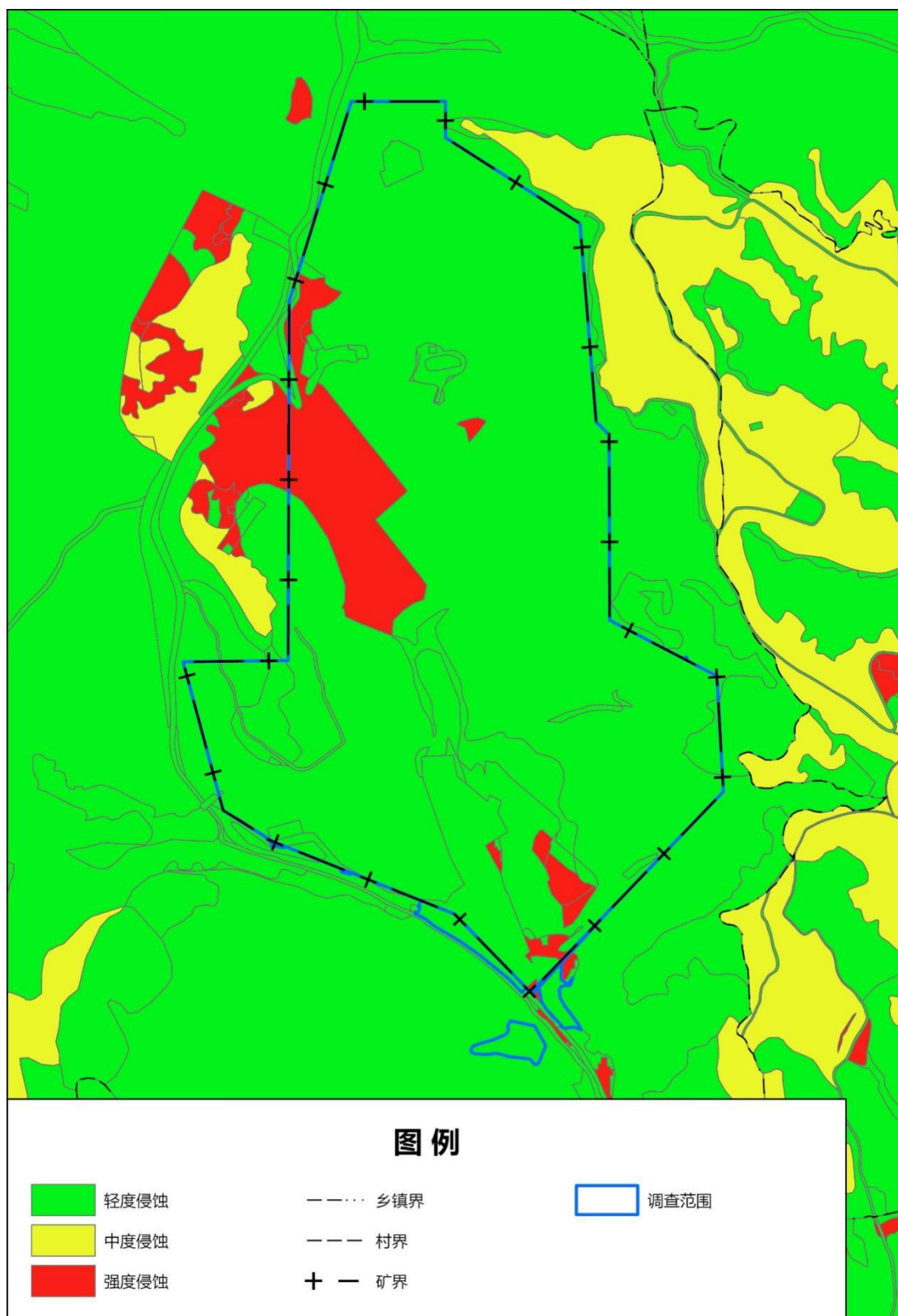
图 2-4-2 调查区土壤侵蚀现状图
