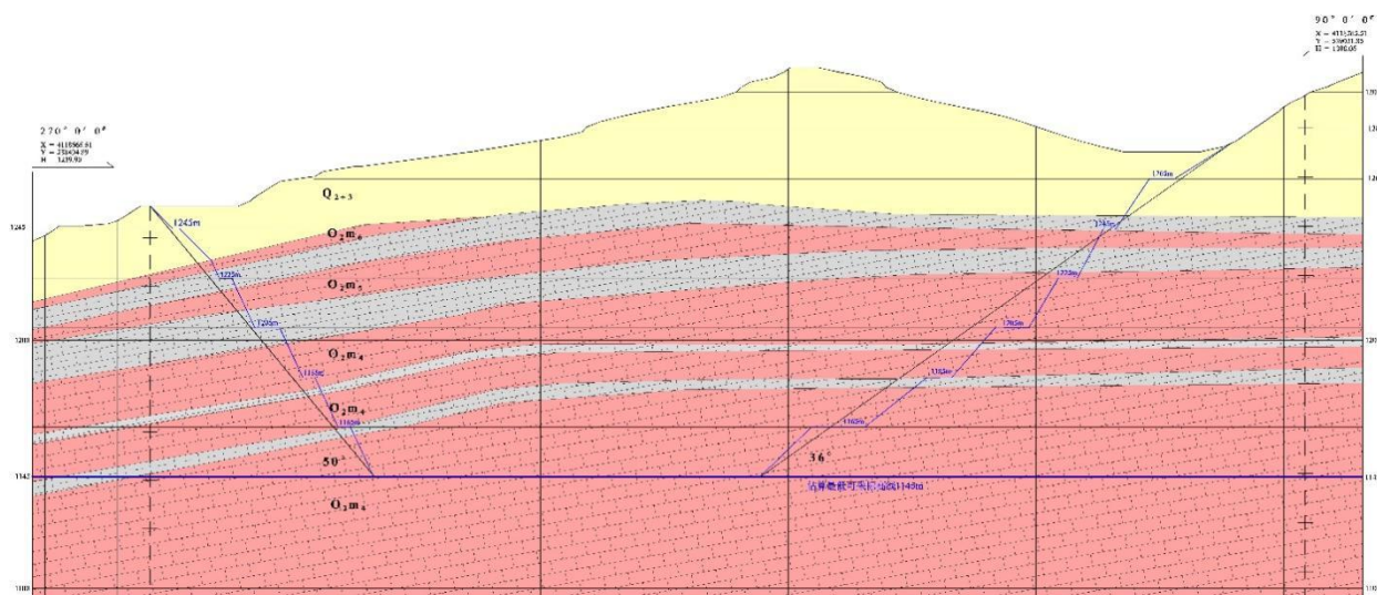
图 8-5 设计露天采场终了边坡剖面图
