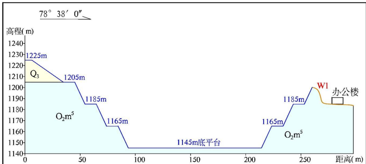
图 8-6 工业场地挖方边坡 W1 剖面图
