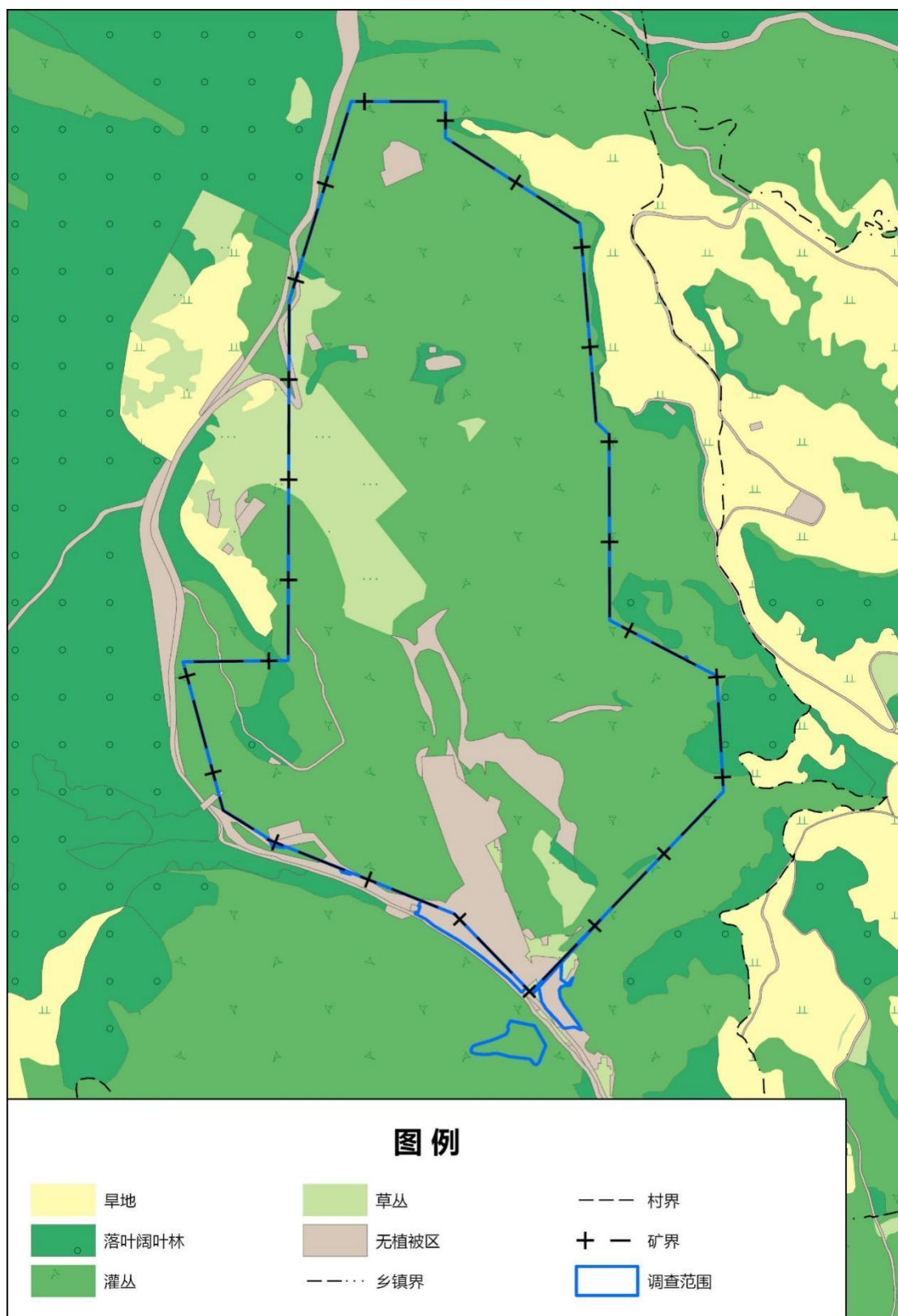
图 2-4-1 调查区植被类型图
