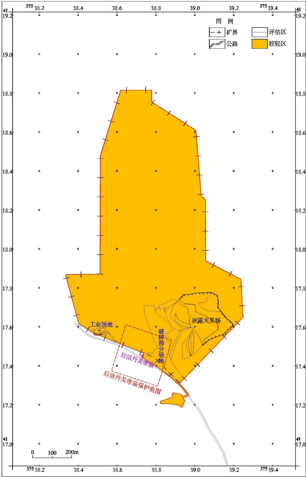
图 8-2 地质灾害现状评估图
