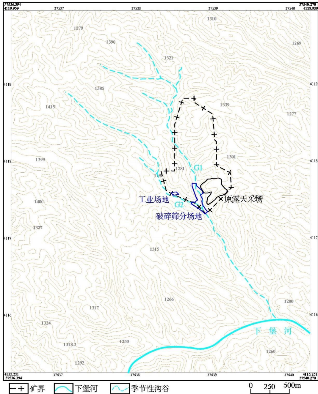
图 2-1 矿区水系图
