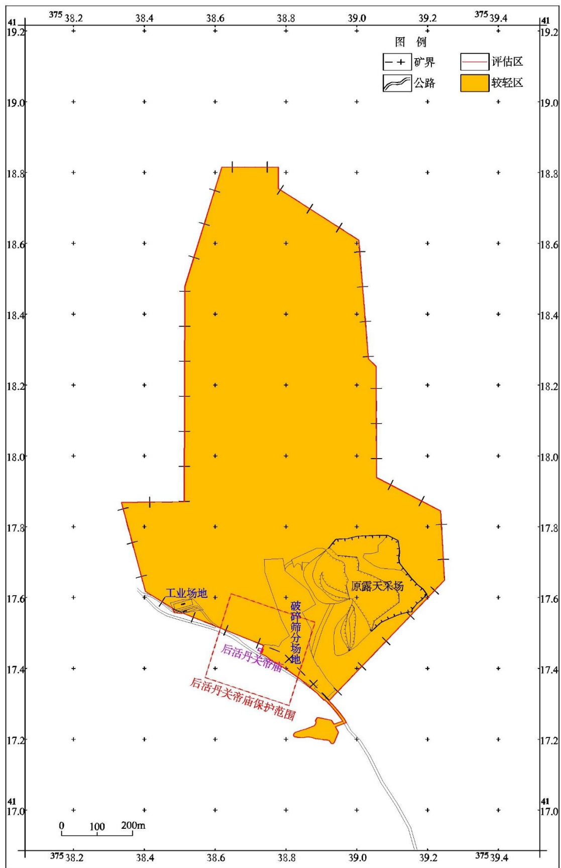
图 8-3 含水层影响或破坏程度现状评估图
