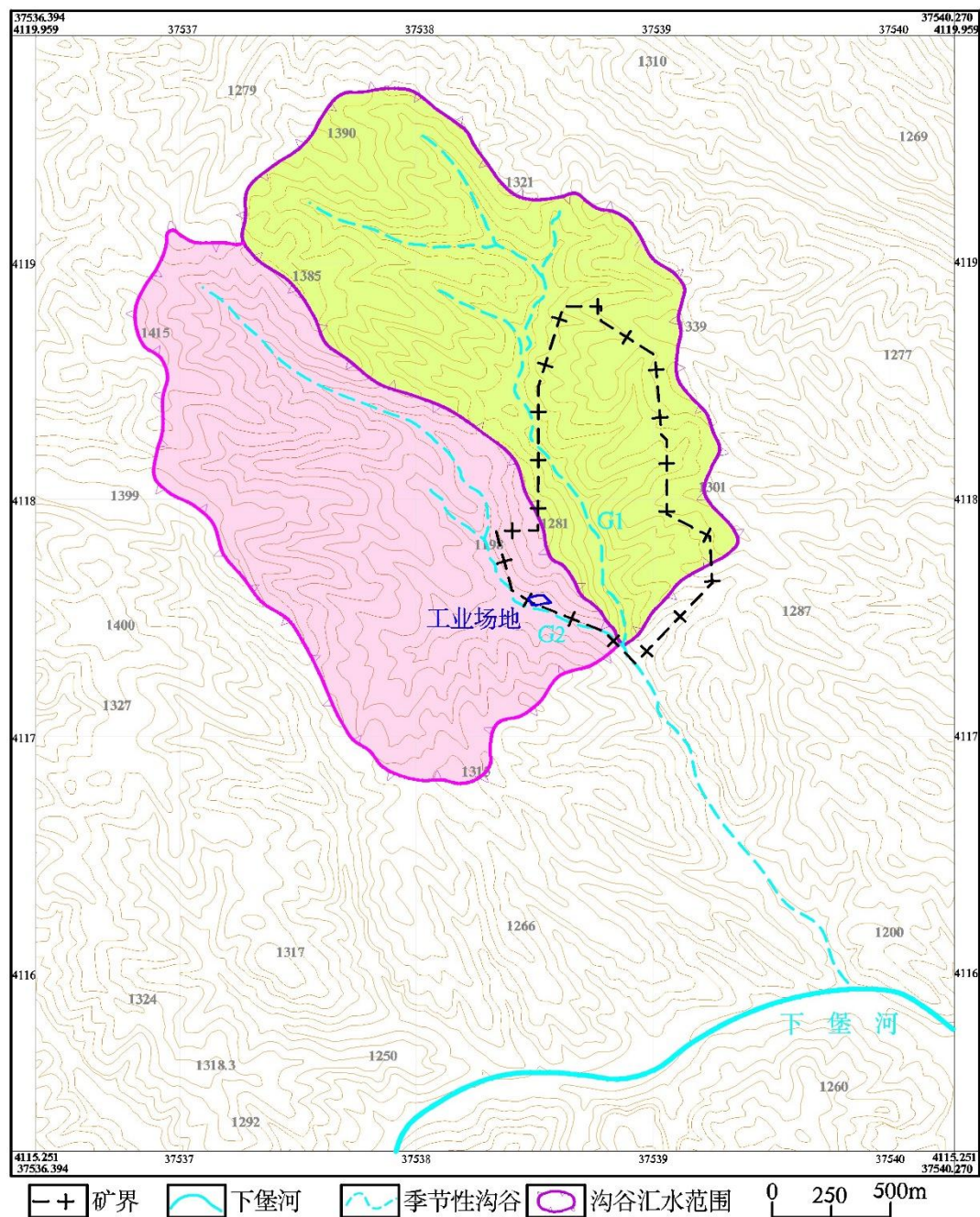
图 8-6 沟谷汇水范围图
