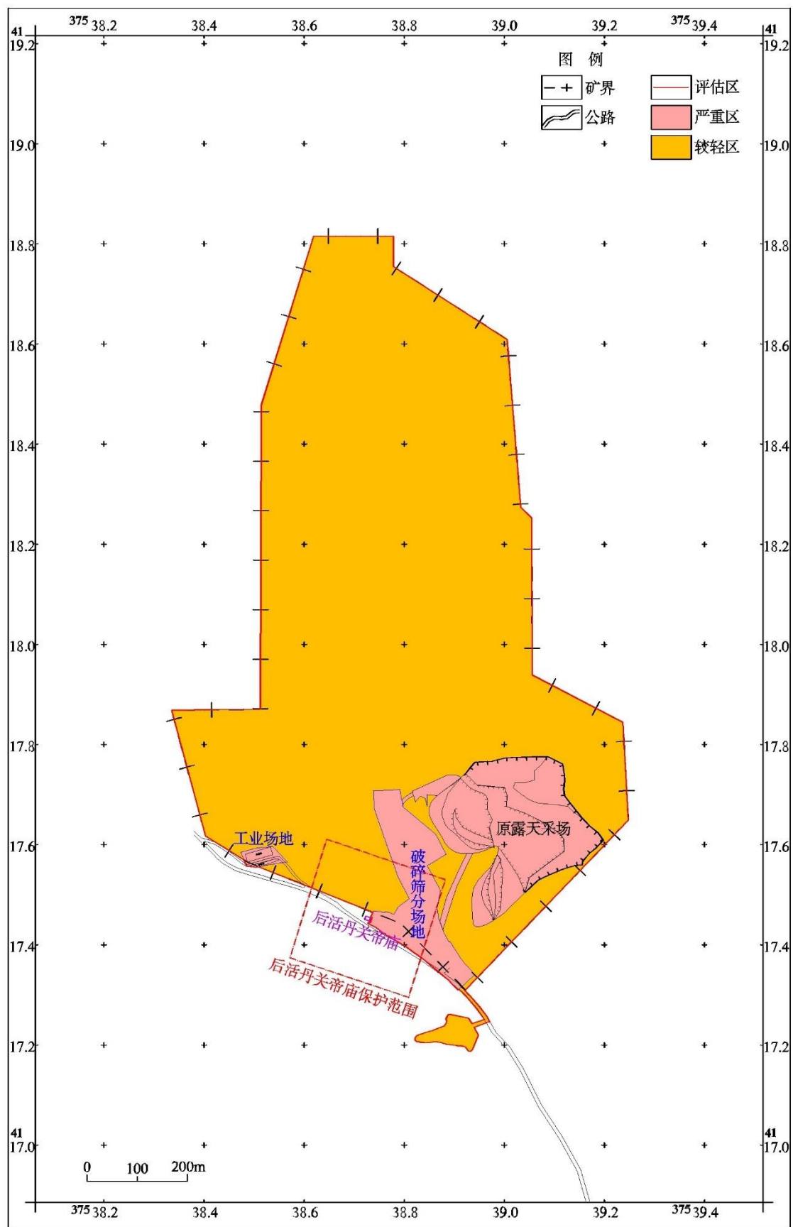
图 8-4 地形地貌景观影响和破坏程度现状评估图
