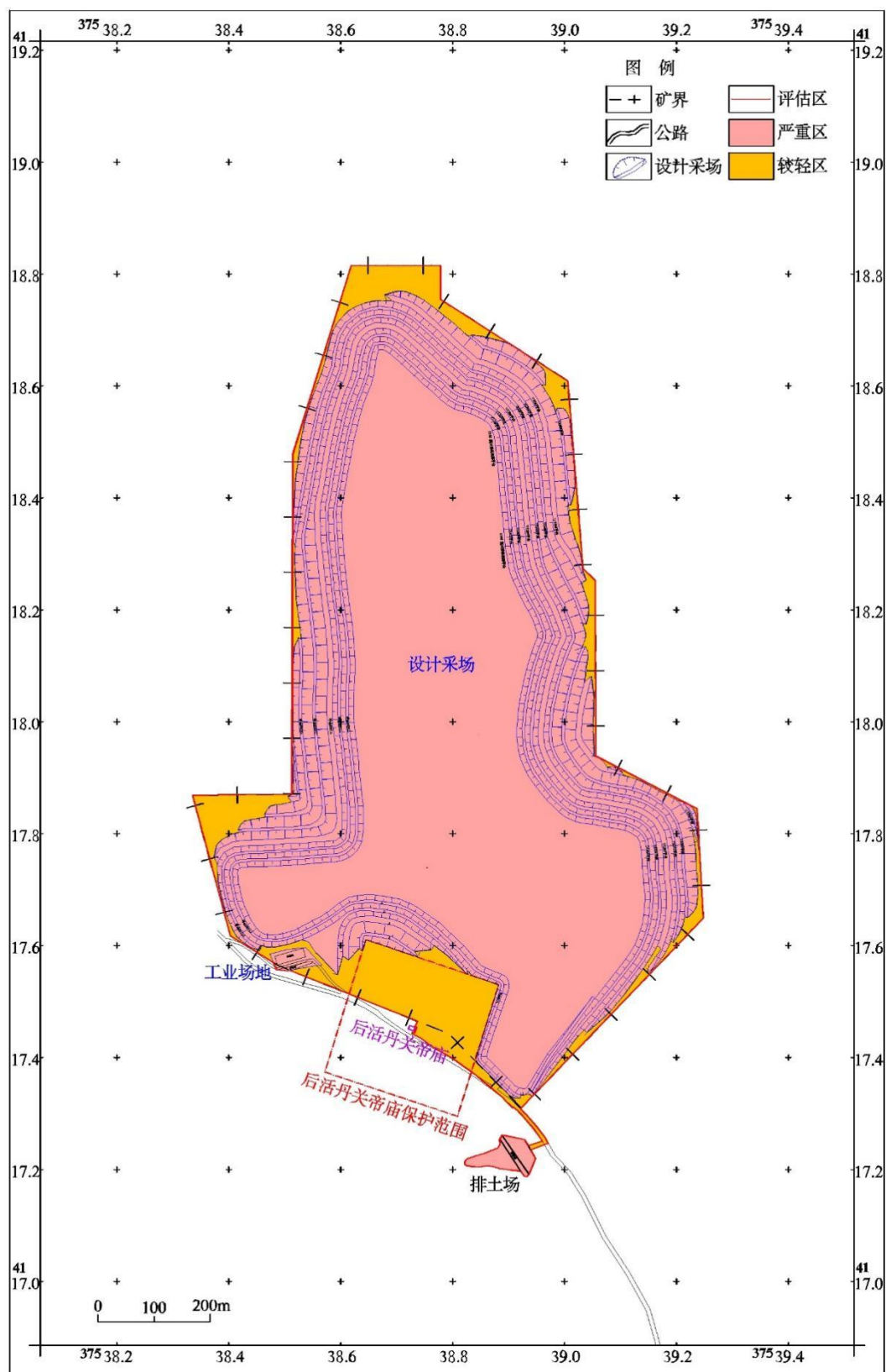
图 8-9 地形地貌景观影响与破坏预测评估图
