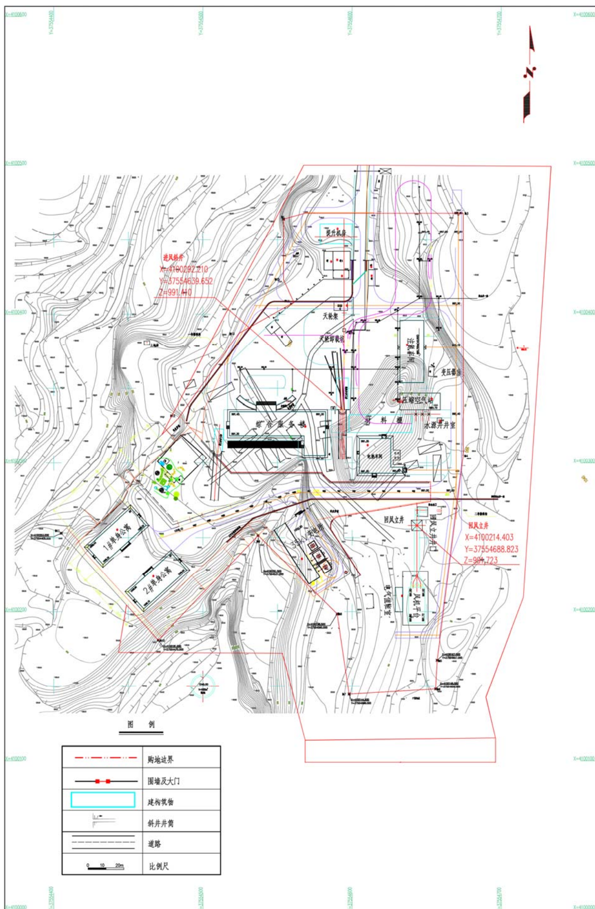
图 3.1-17 后河工业场地平面布置图
