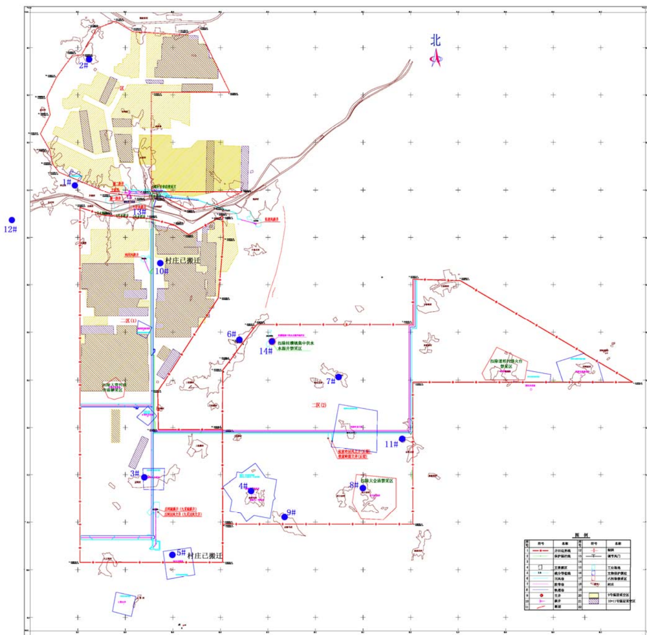
图 3.1-19 水井与采空区分布图
