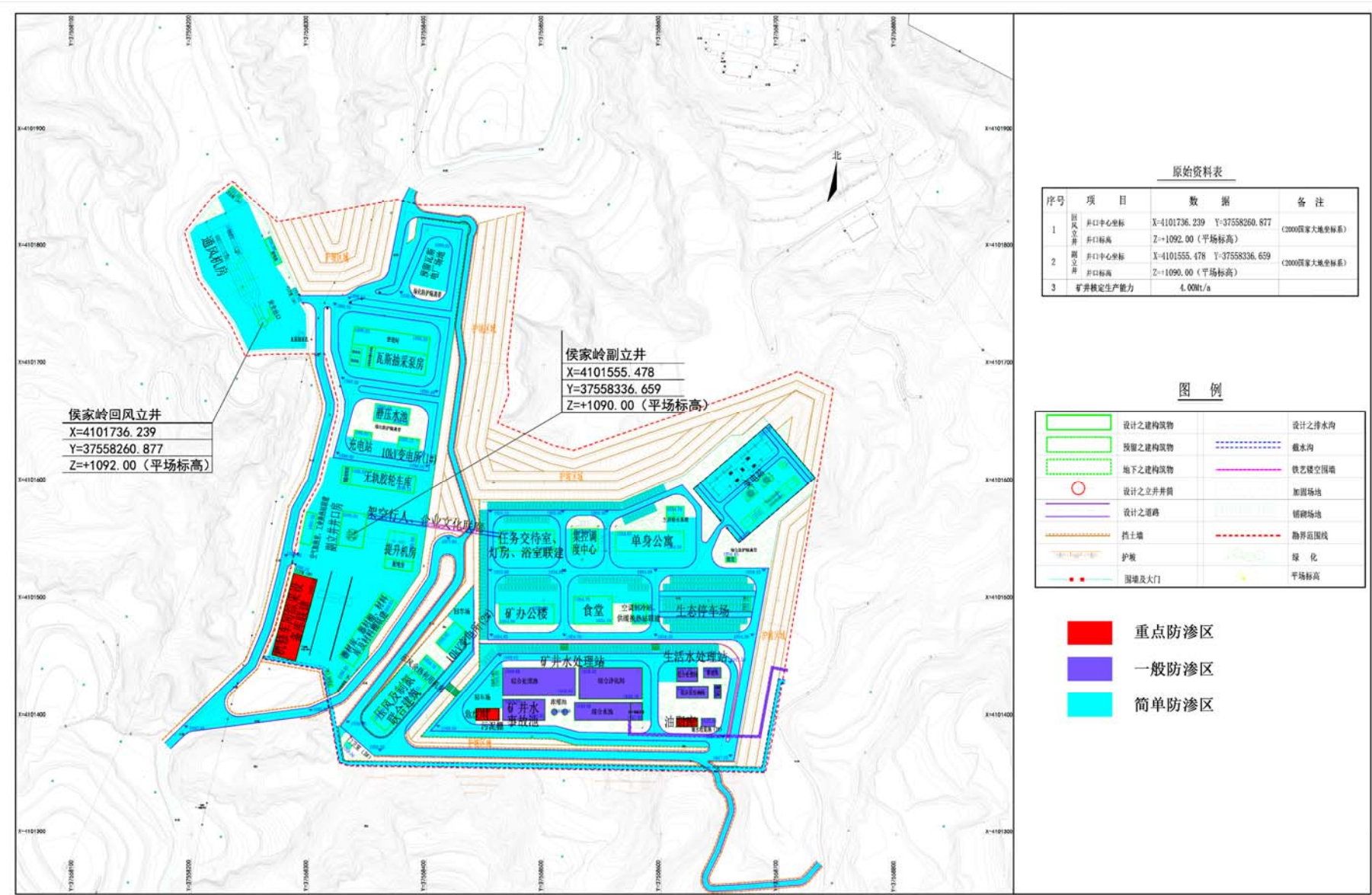
图 6.2-3 分区防渗图
