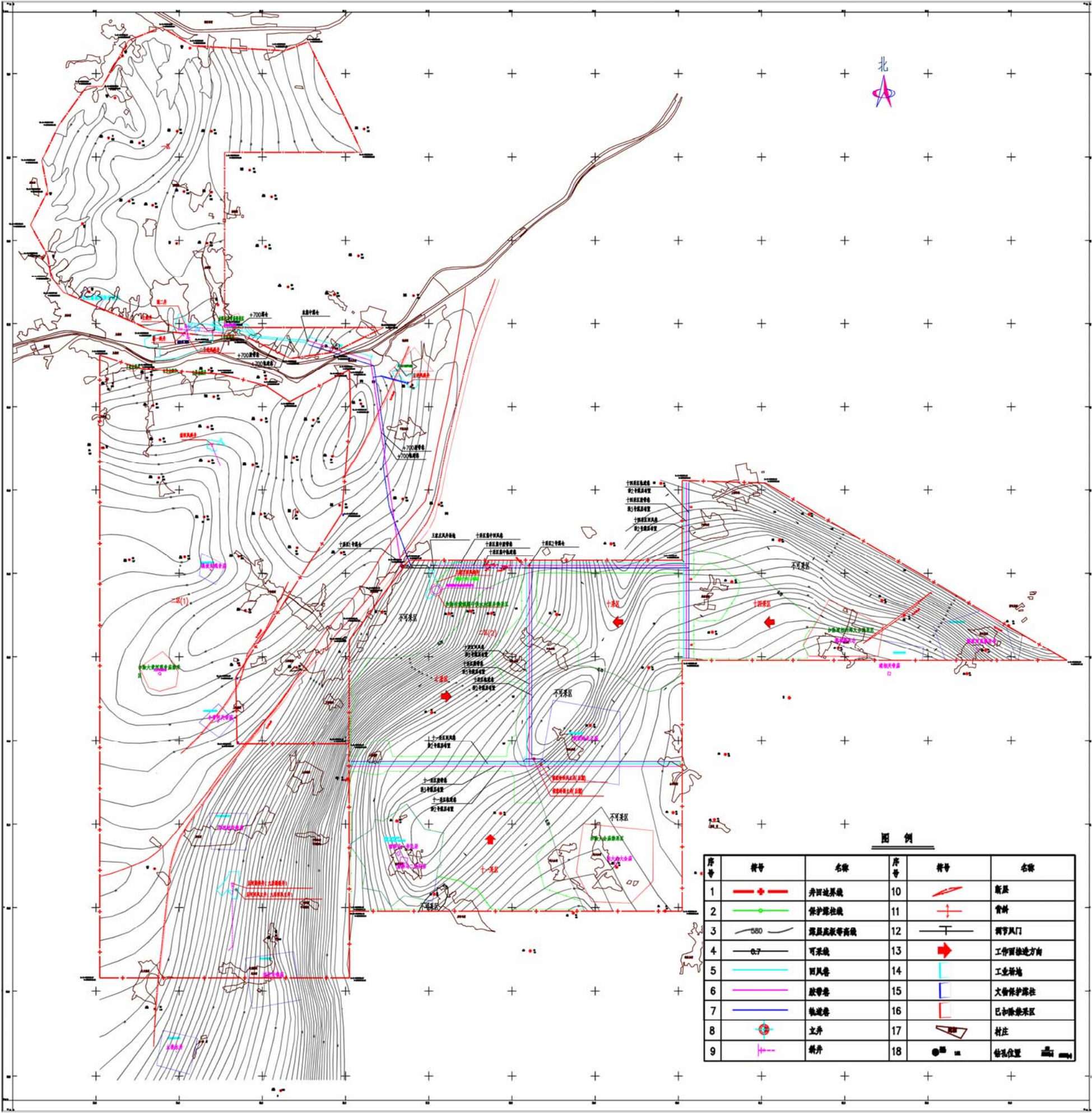
图 3.1-2 3 号煤层采掘布置图
