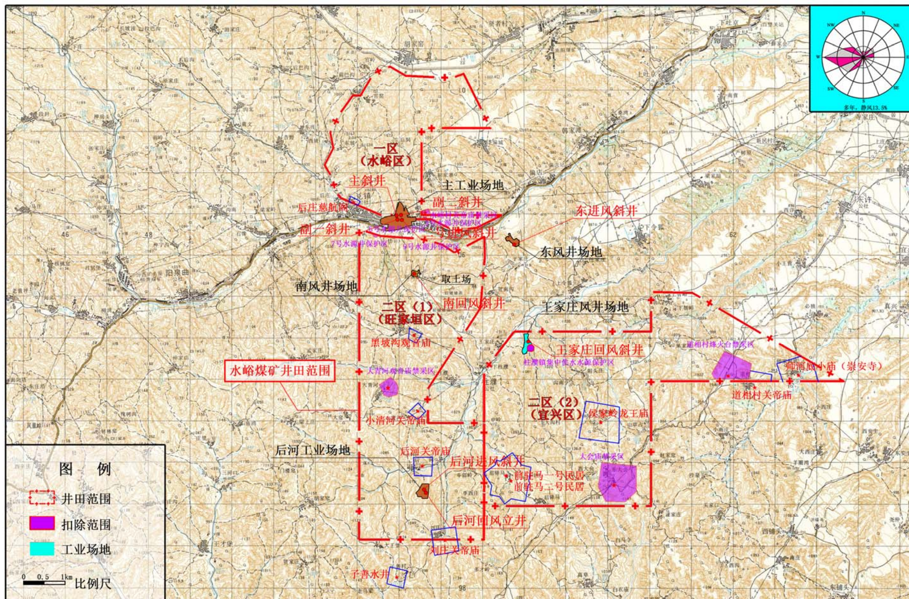
图 3.1-13 现有工程总平面布置图
