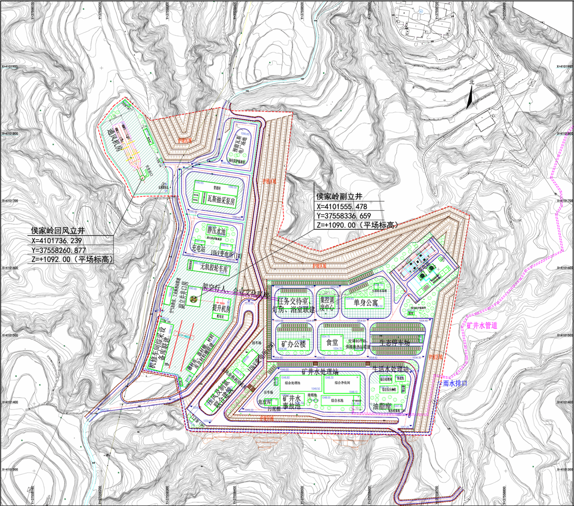
图 3.2-7 侯家岭场地平面布置
