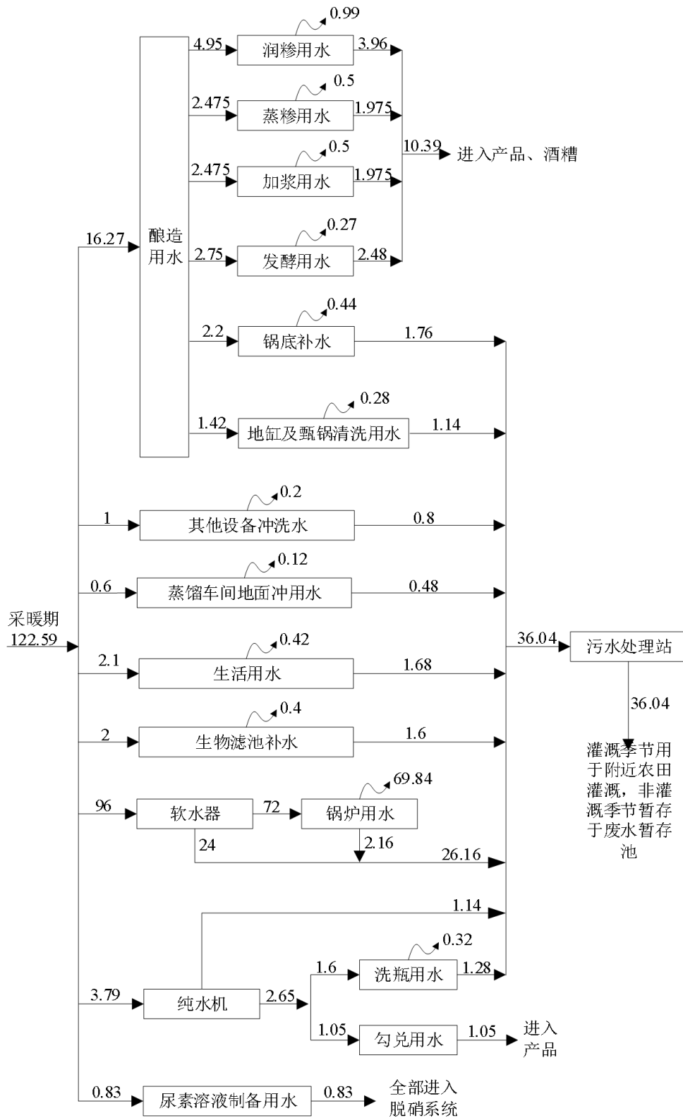
图 3.3-1 本项目采暖期水平衡图 (m³/d)
