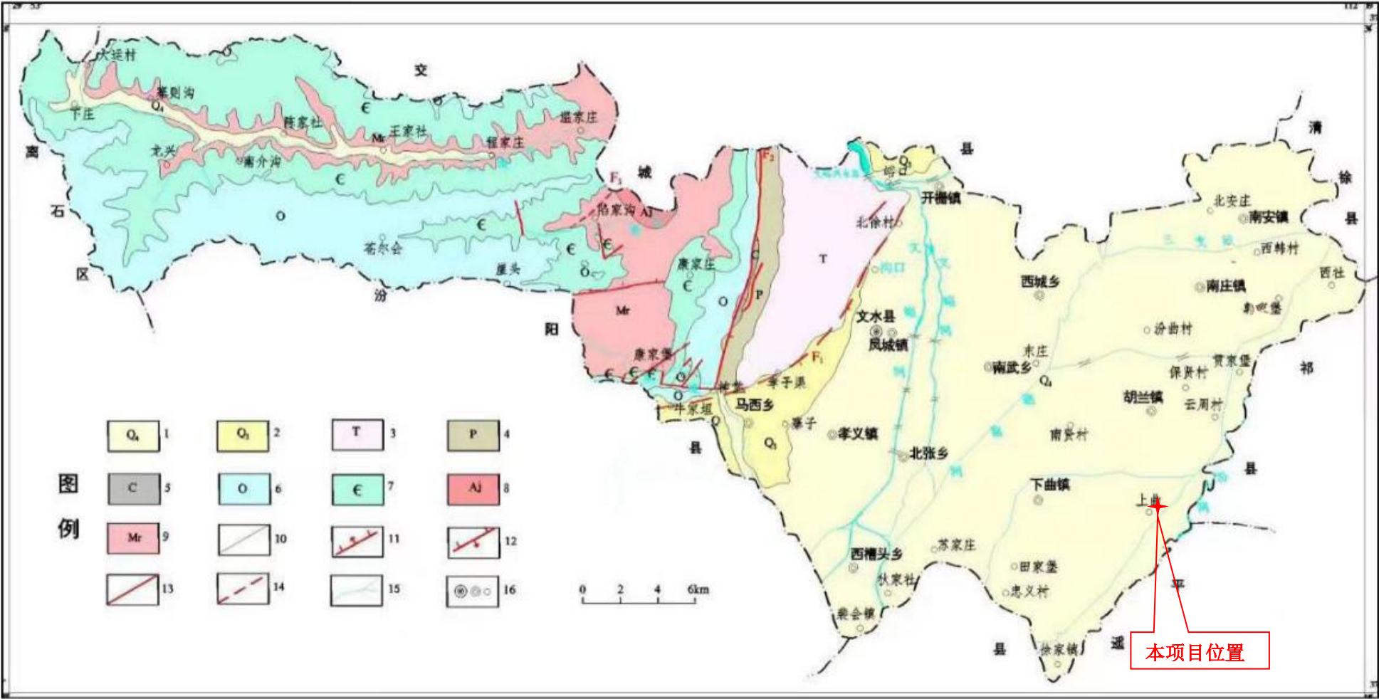
图 4.1-6 项目评价区地质图
