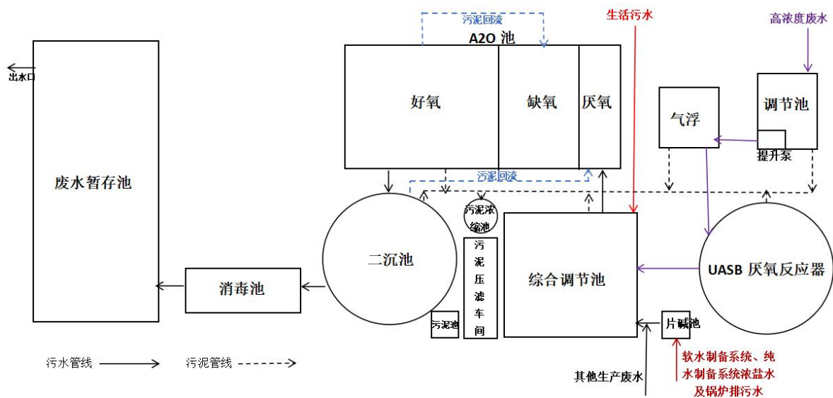
图 6.2-3 污水处理站平面布置示意图
