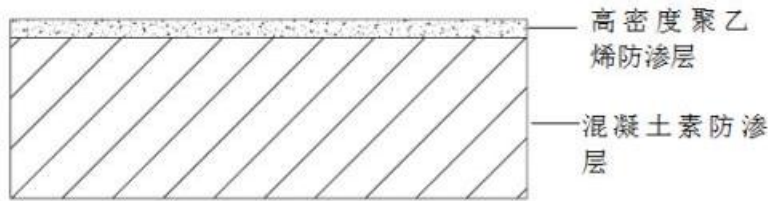
图 5.4-1 危废贮存点防渗层剖面图
