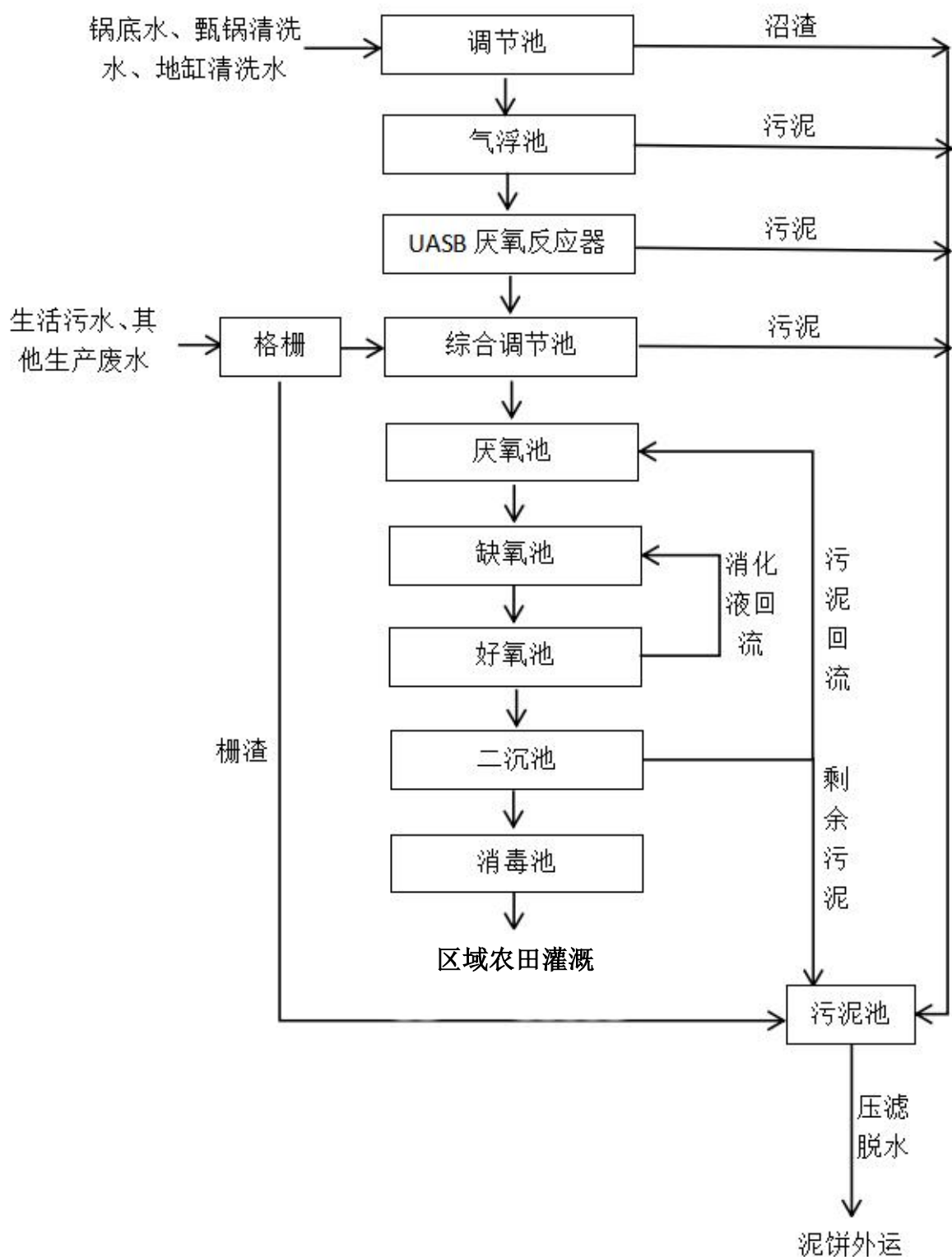
图 6.2-2 污水处理站工艺流程图
