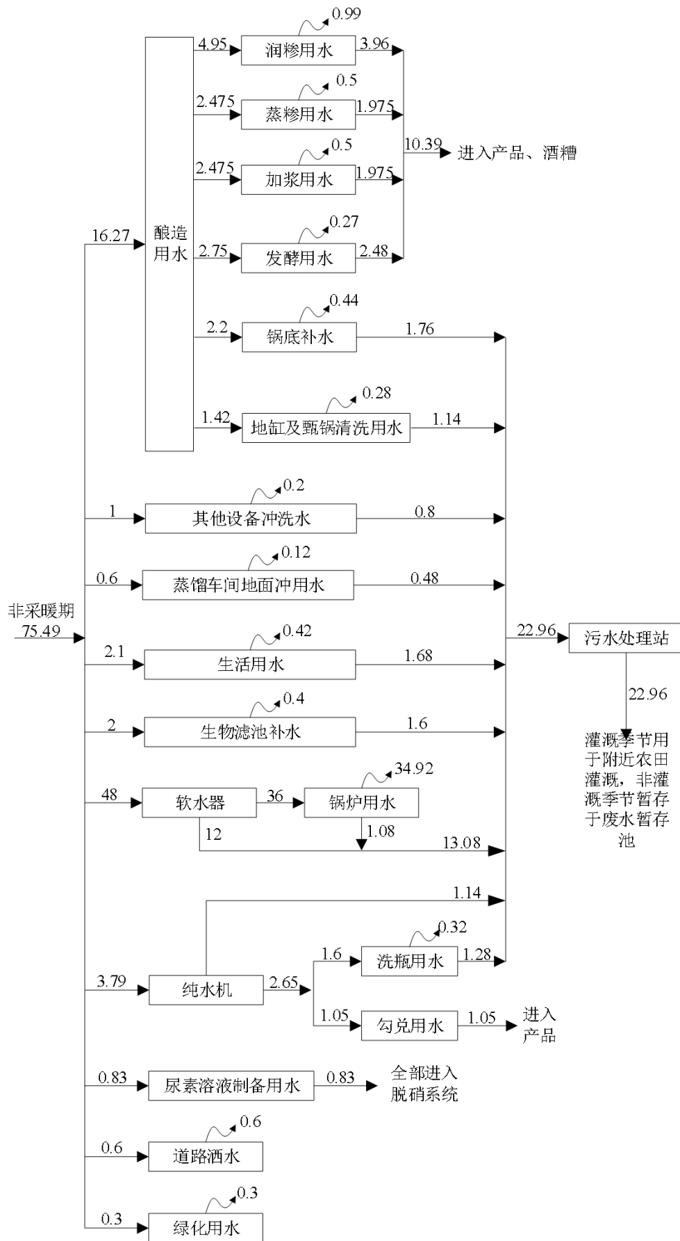
图 3.3-2 本项目非采暖期水平衡图 ( \text{m}^3/\text{d} )
