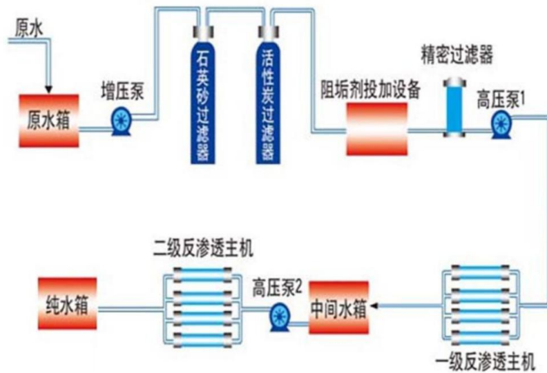
图 3.4-2 纯水制备工艺流程图
