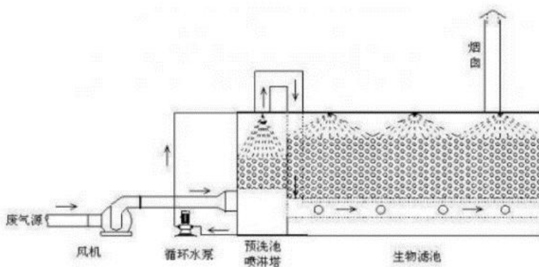
图 6.2-1 生物滤池除臭流程图
