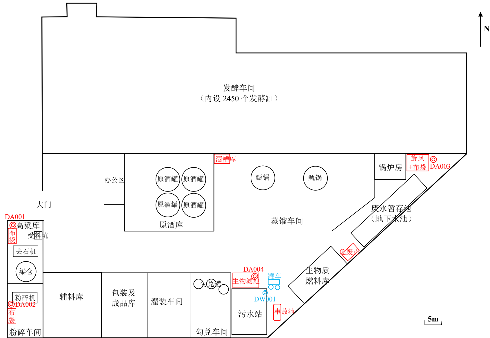
图 3.2-1 本项目厂区平面布置图
