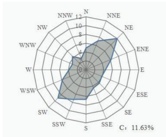
图 5.1-1 全年风向频率玫瑰图
