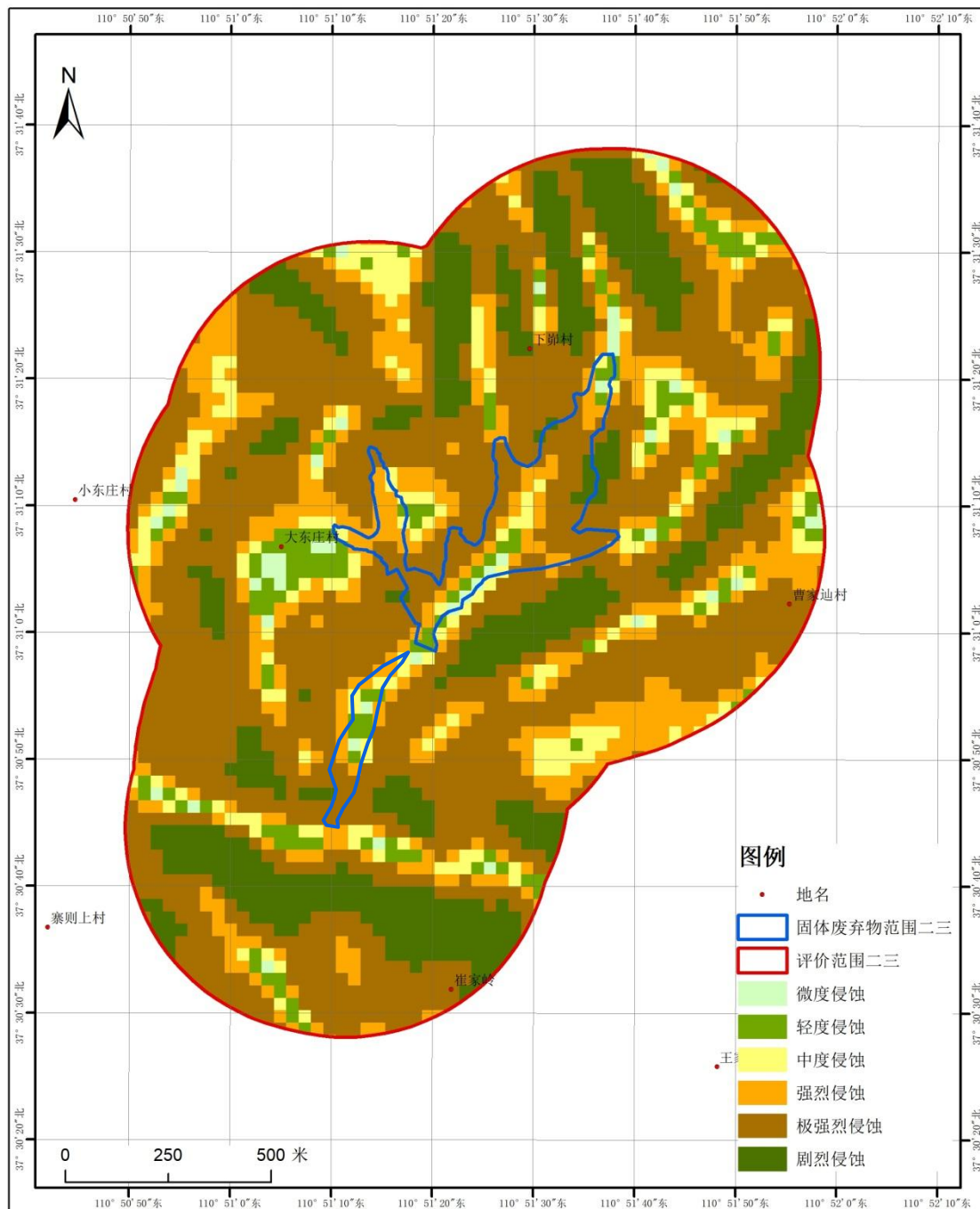
图 4.3.5-3 大东庄土壤侵蚀现状图
