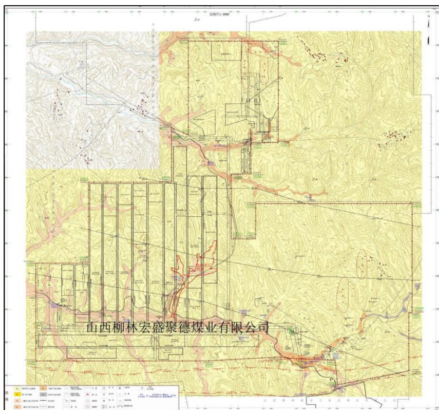
图 3.3-2 (b) 大东庄场区（地块二）与 8#煤层采空区关系位置图
