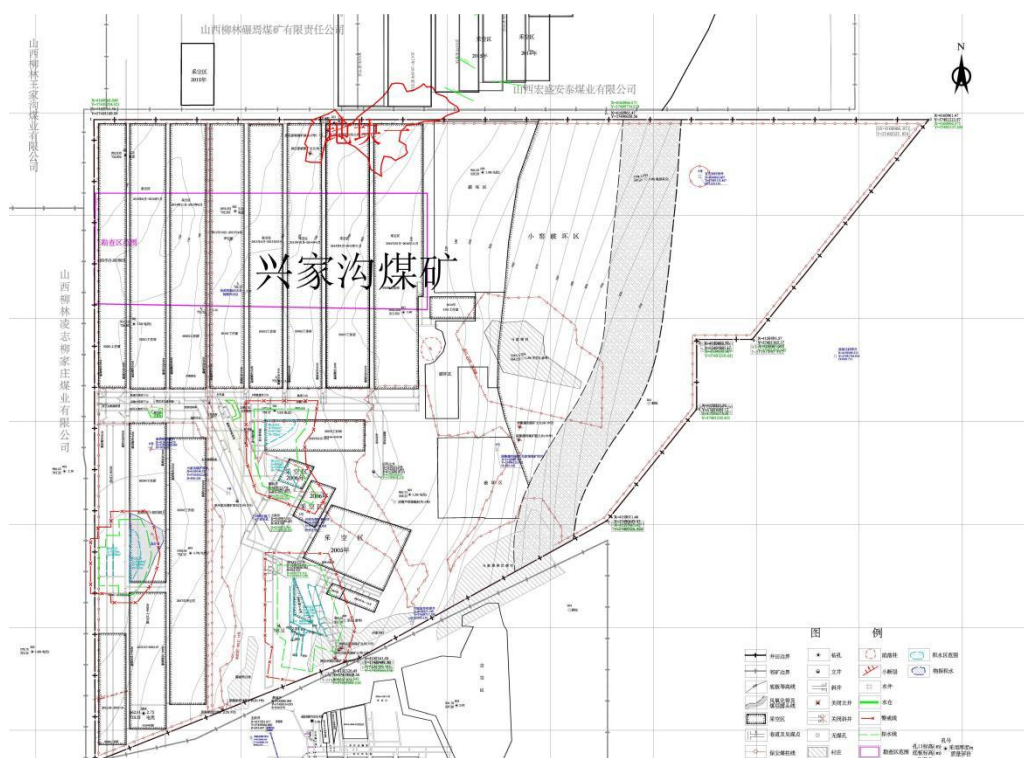
图 3.3-1 (b) 田家坡场区（地块一）与 8#煤层采空区关系位置图
