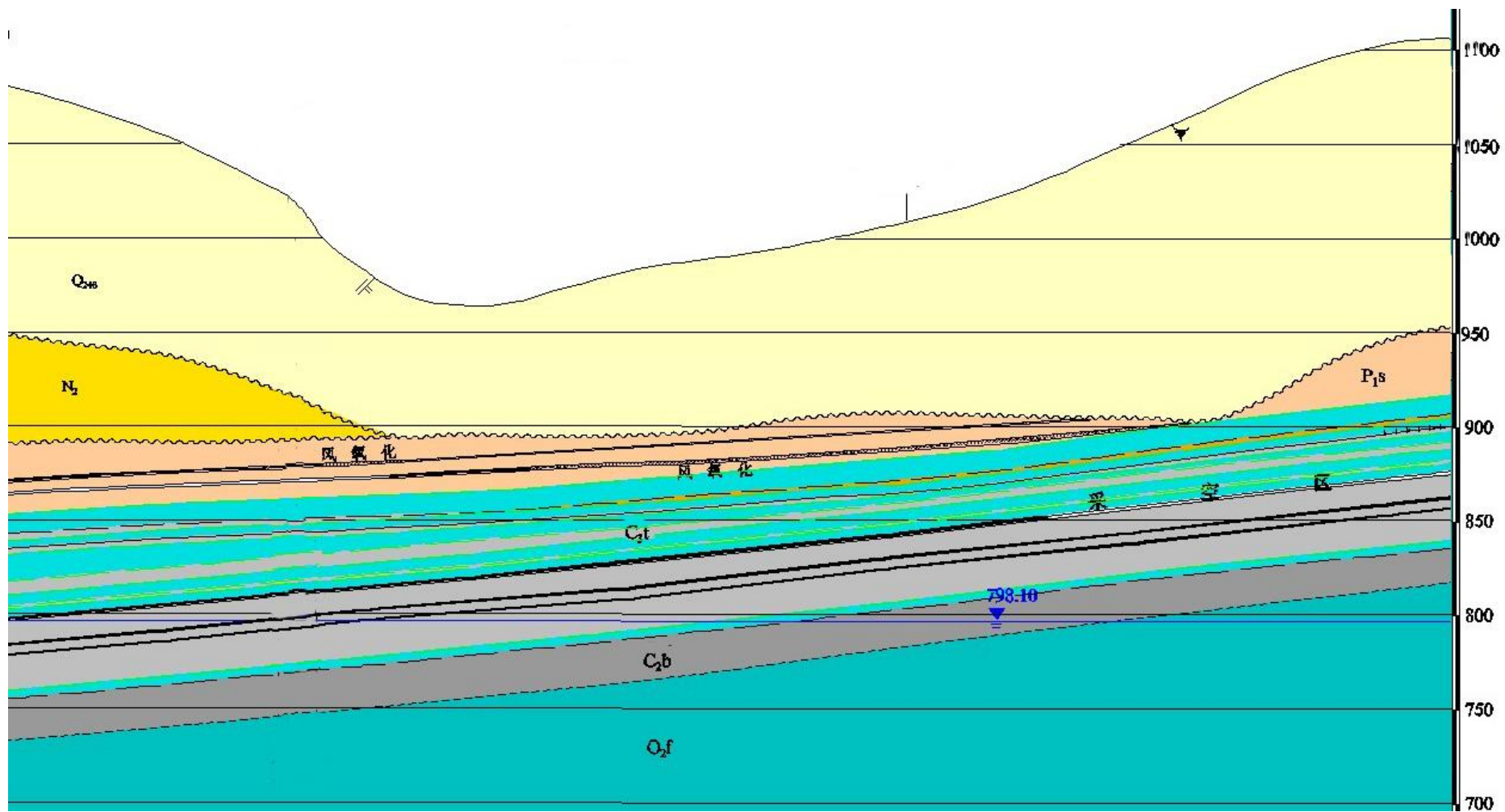
图 4.1-7 田家坡水文地质剖面图 1-1'
