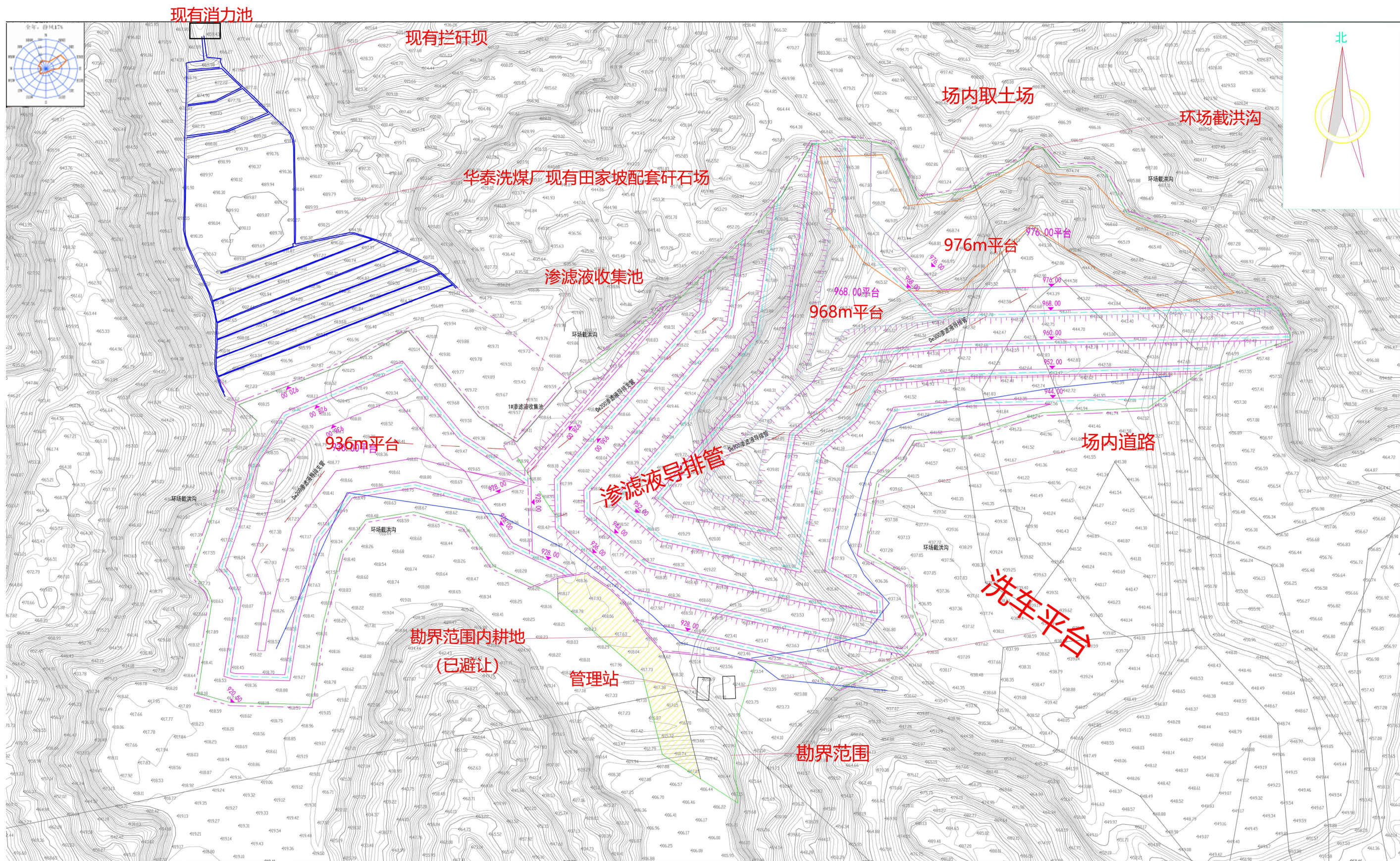
图 3.3-1 田家坡场区平面布置图
