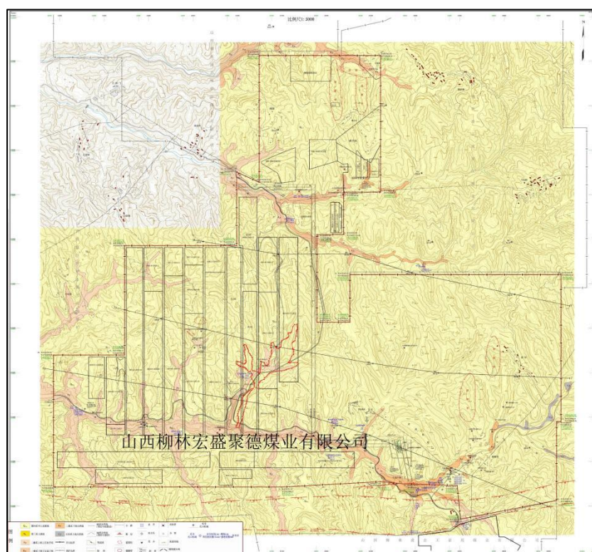
图 3.3-2 (c) 大东庄场区（地块二）与 9#煤层采空区关系位置图
