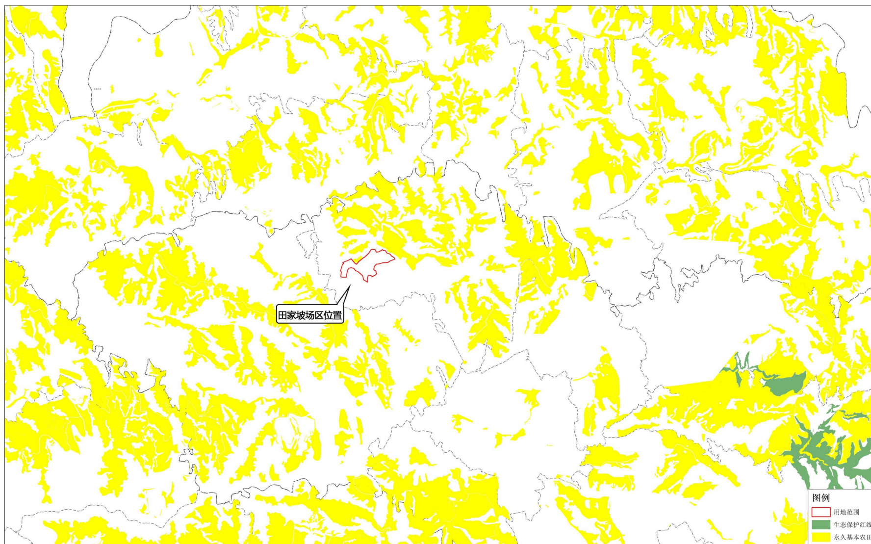
图 2.6-1 田家坡场区与柳林县“三区三线”位置关系图
