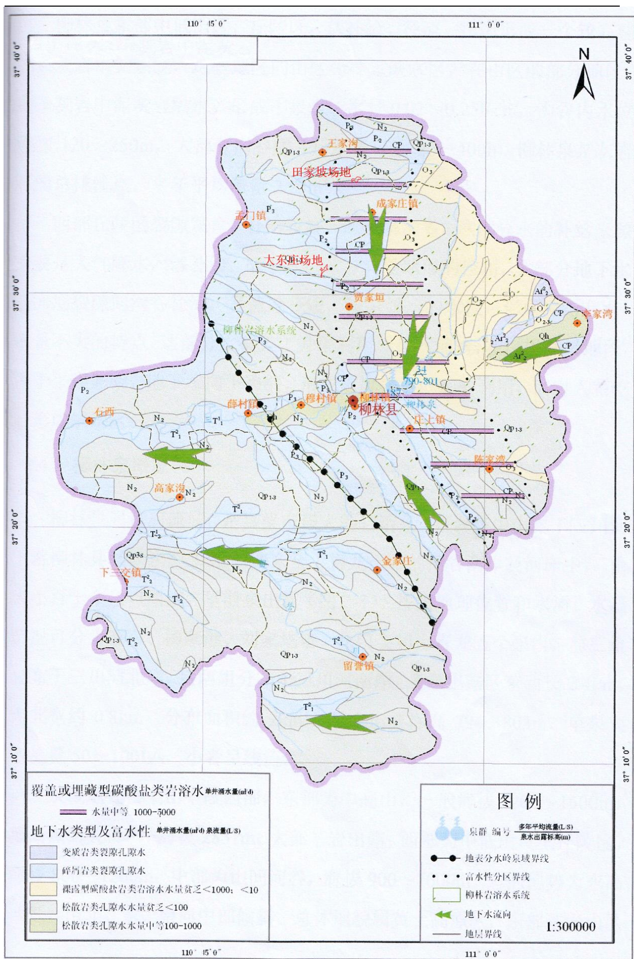
图 4.1-5 区域水文地质图
