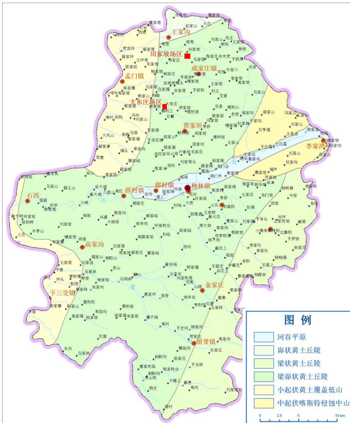
图 4.1-3 柳林县地形地貌图
