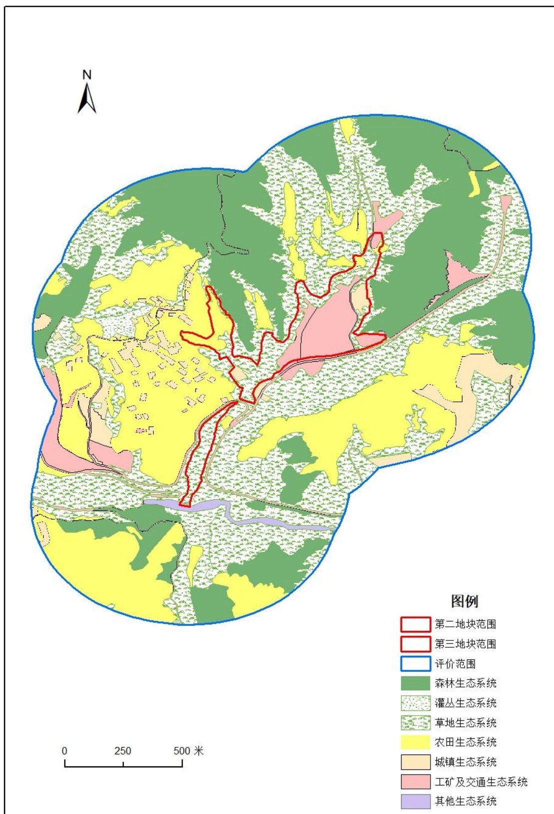
图 4.3.5-4 大东庄生态系统现状图
