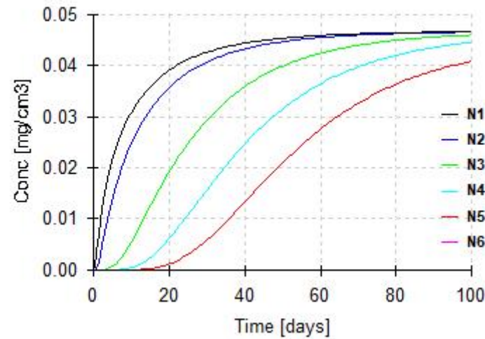
图 5.3-1 镍在不同时间的浓度分布图
