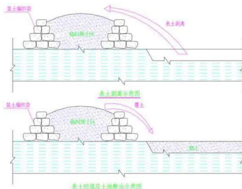
图 3.4-6 表土剥离示意图
