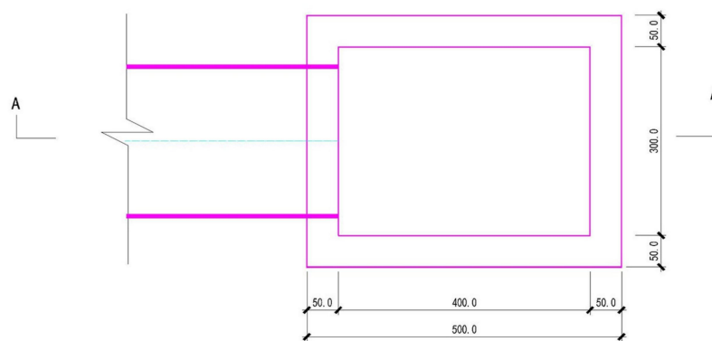
集水池平面图
