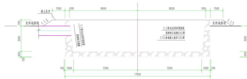
2-2剖面图 1:100
