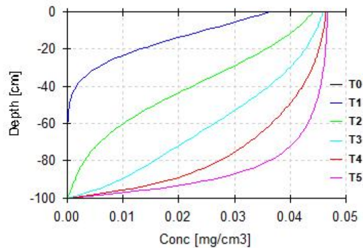
图 5.3-2 不同深度处镍浓度随时间变化曲线
