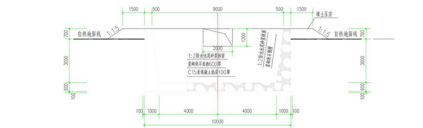
1-1剖面图 1:100
