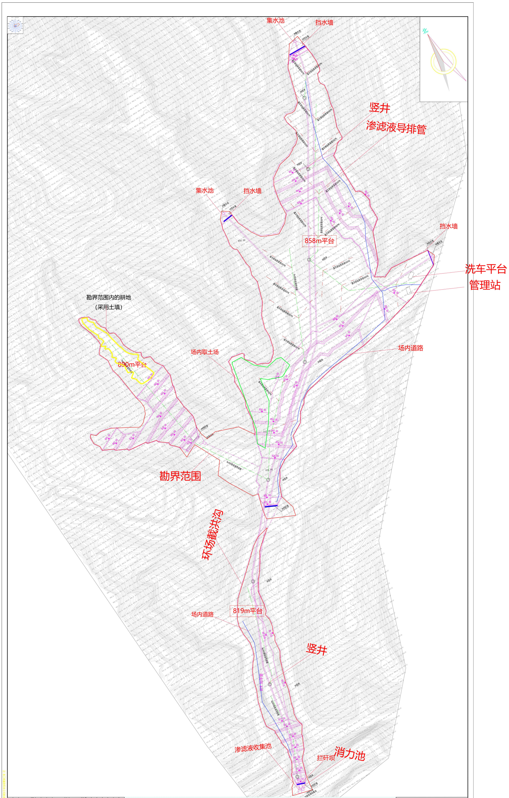
图 3.3-2 大东庄场区平面布置图
