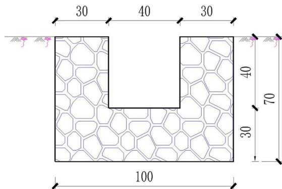
横向排水断面图
