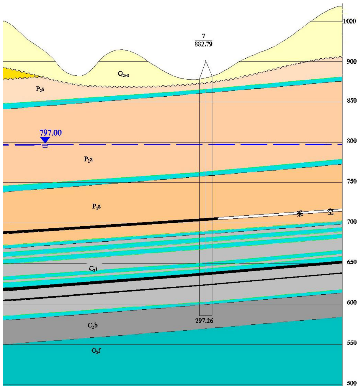
图 4.1-9 大东庄水文地质剖面图
