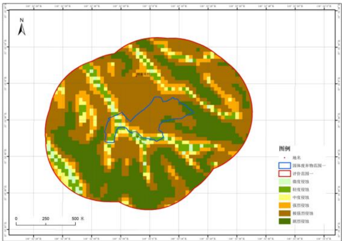
图 4.3.5-3 田家坡土壤侵蚀现状图
