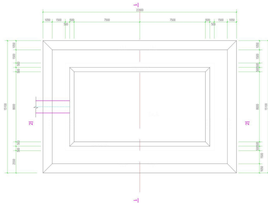
收集澄清池平面布置图 1:100
