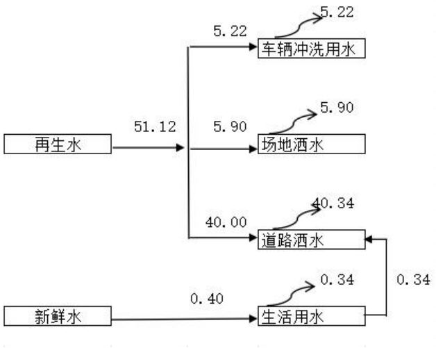
图 3.2-5 项目回填作业期水平衡图（m 3 /d）
