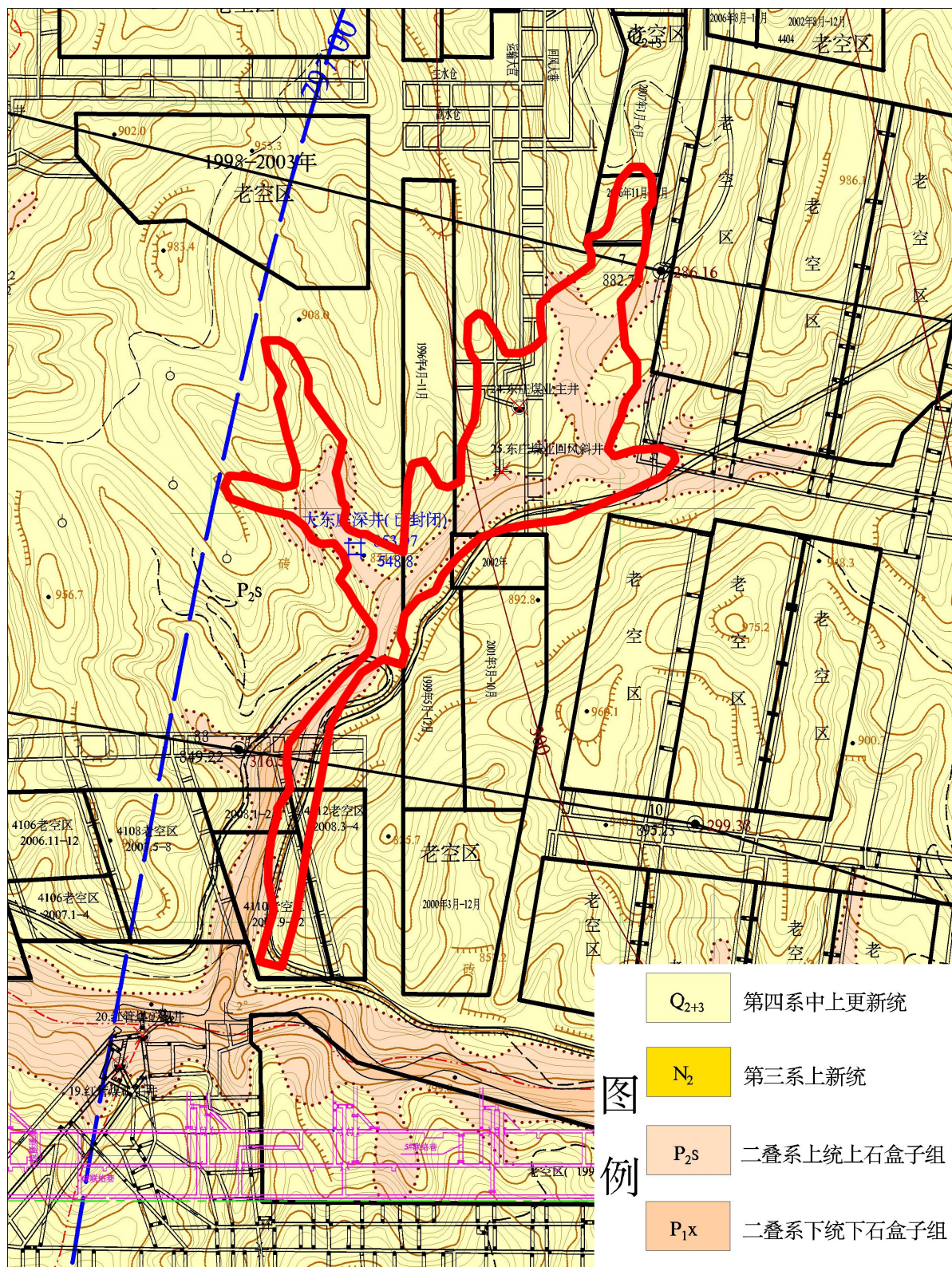
图 4.1-8 大东庄水文地质图
