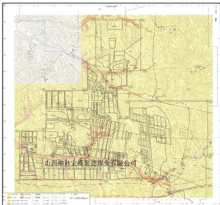
图 3.3-2 (a) 大东庄场区（地块二）与 4#煤层采空区关系位置图
