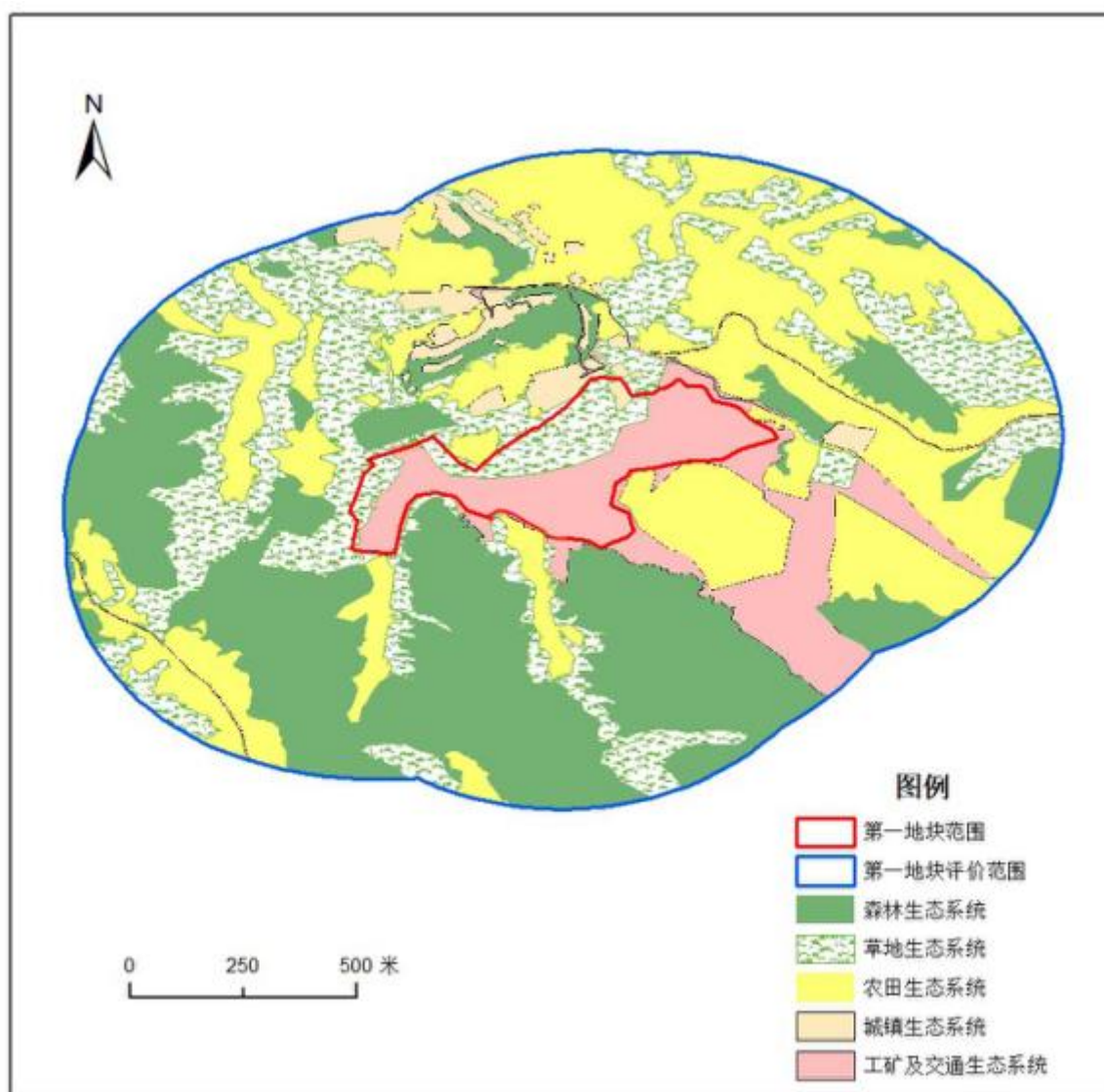
图 4.3.5-4 田家坡生态系统现状图
