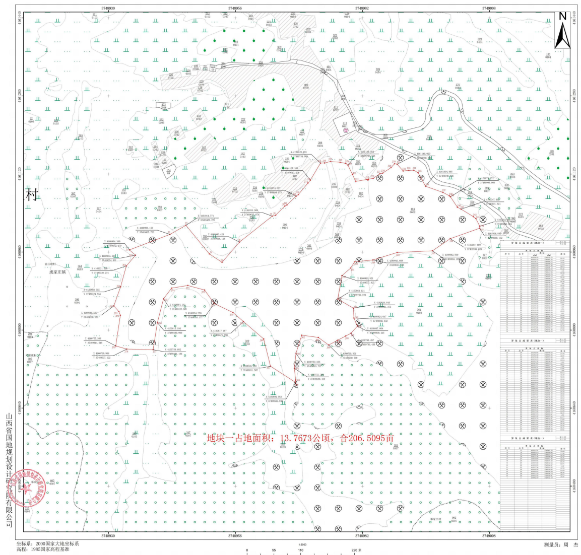
离柳煤基固废生态回填及区域生态修复治理试点项目勘测定界图
