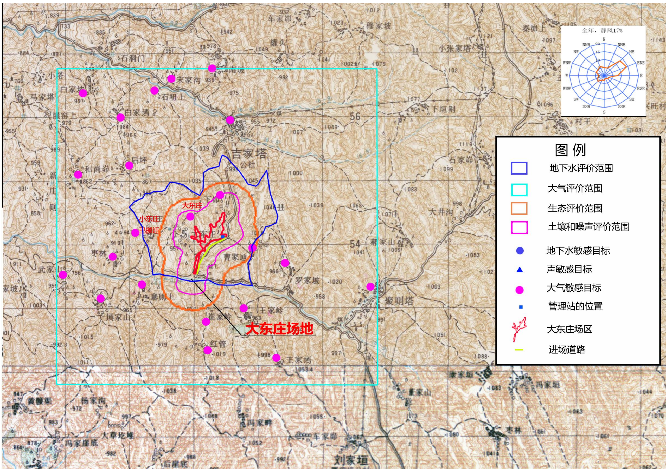
图 2.6-4 本项目大东坡场地地理位置 (1 格 1km)、评价范围及环境敏感目标图
