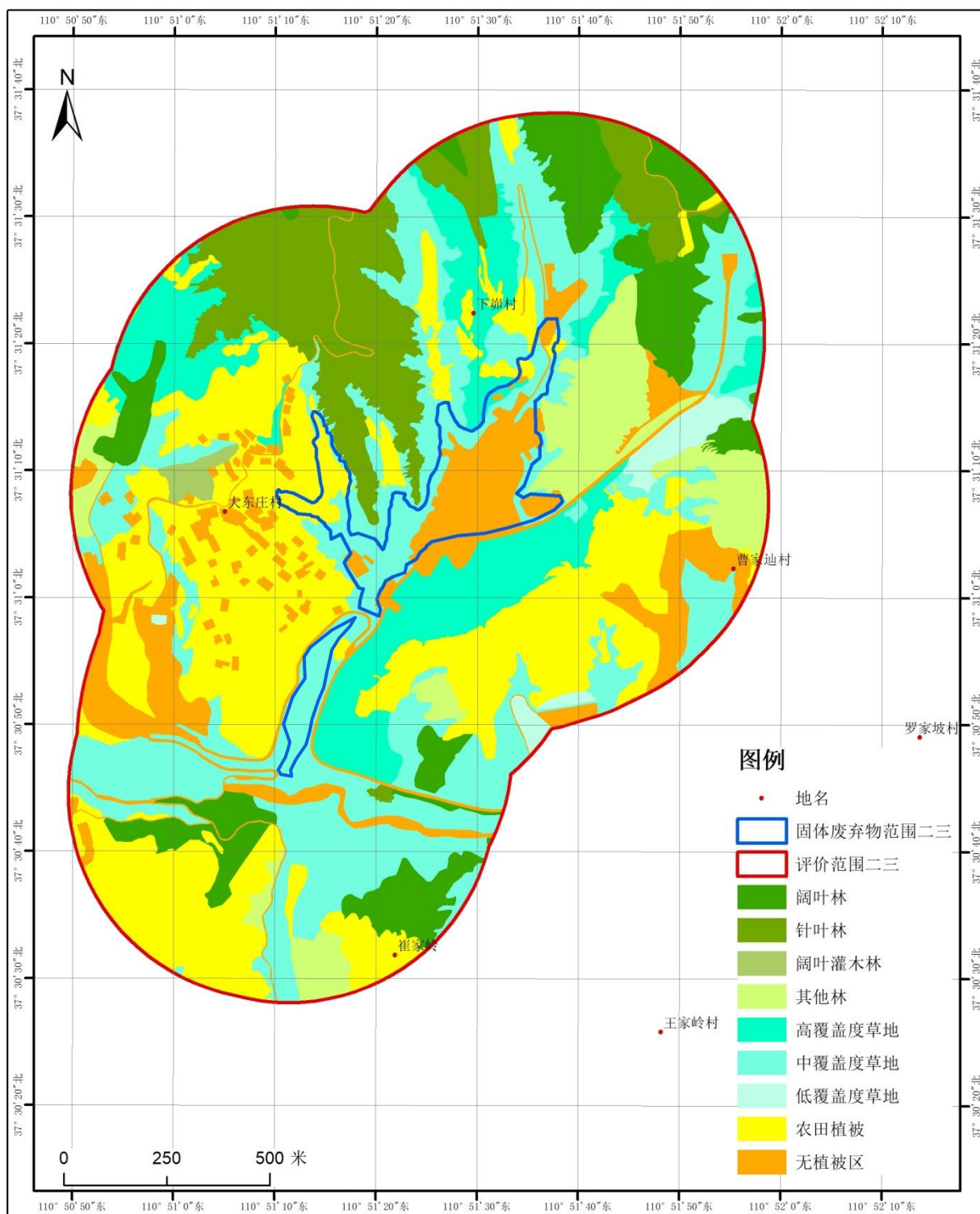
图 4.3.5-2 大东庄地块植被类型现状图
