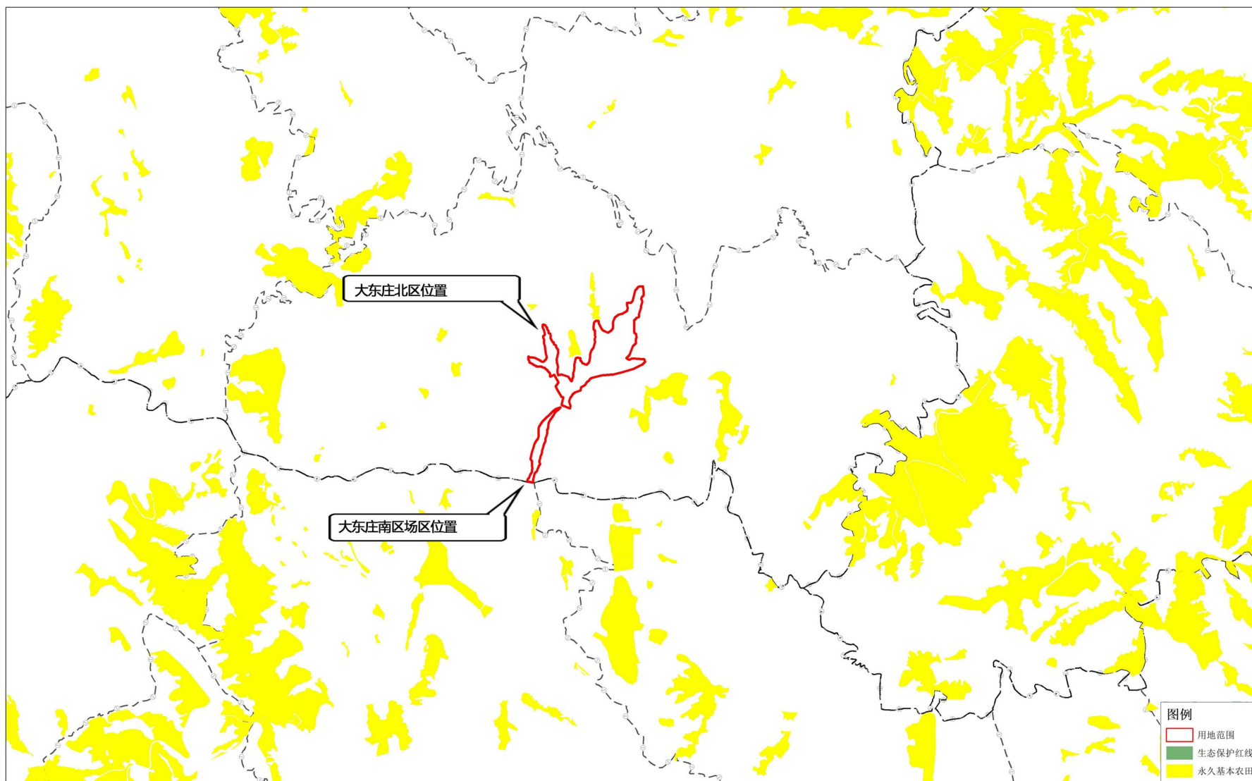
续图 2.6-2 大东庄场区与柳林县“三区三线”位置关系图
