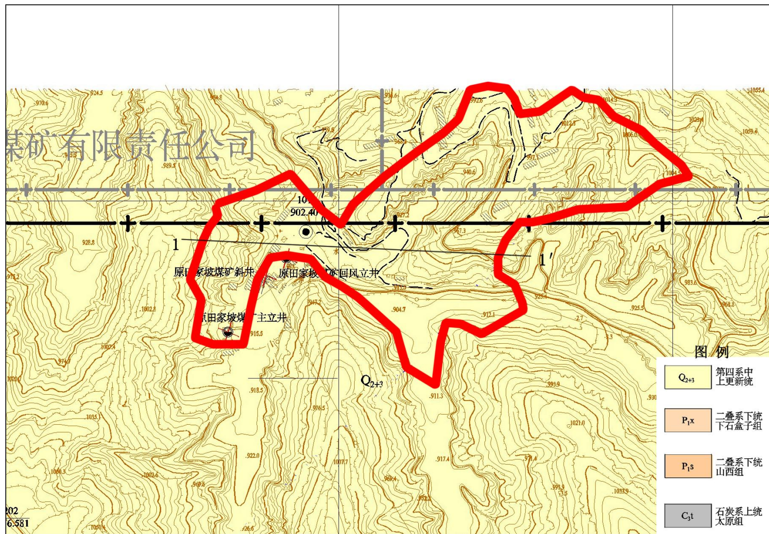
图 4.1-6 田家坡水文地质图
