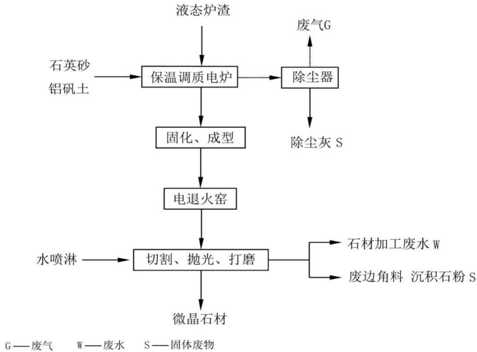
图 3.1-7 微晶石材生产工艺流程图
