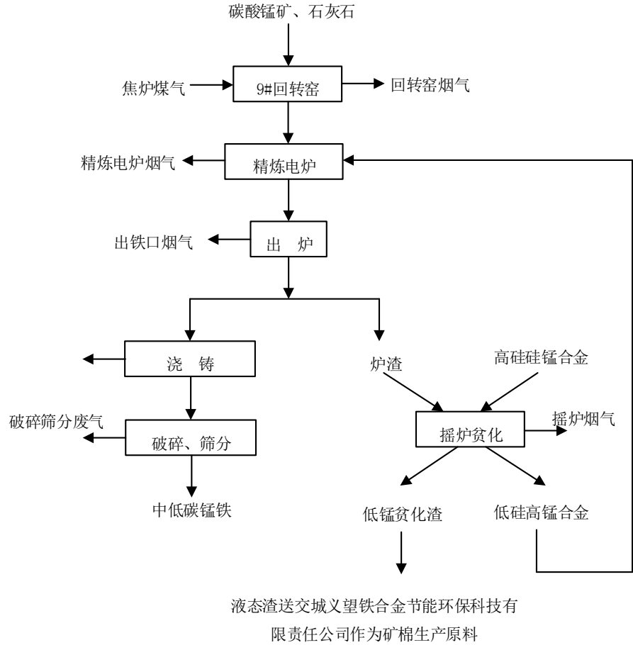
图 3.1-1 一车间生产工艺流程图
