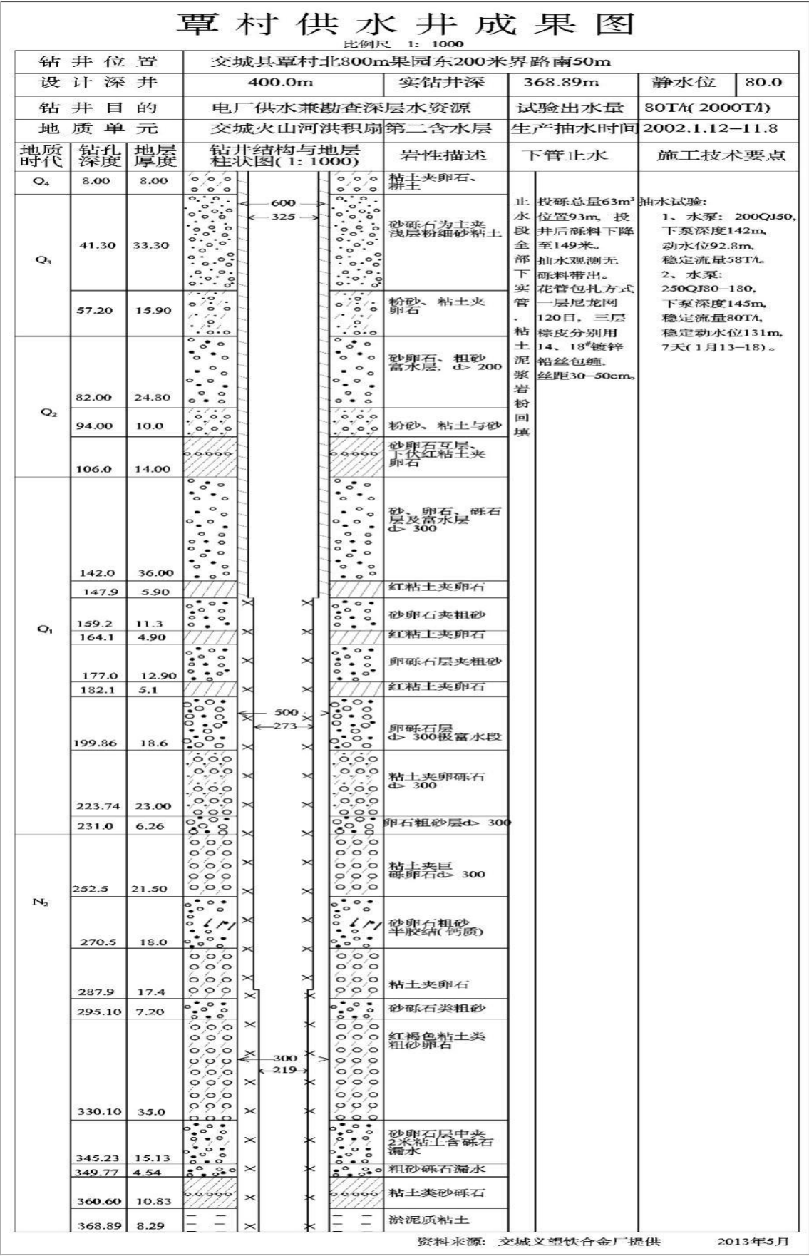
图 5.3-4 覃村供水井成果图
