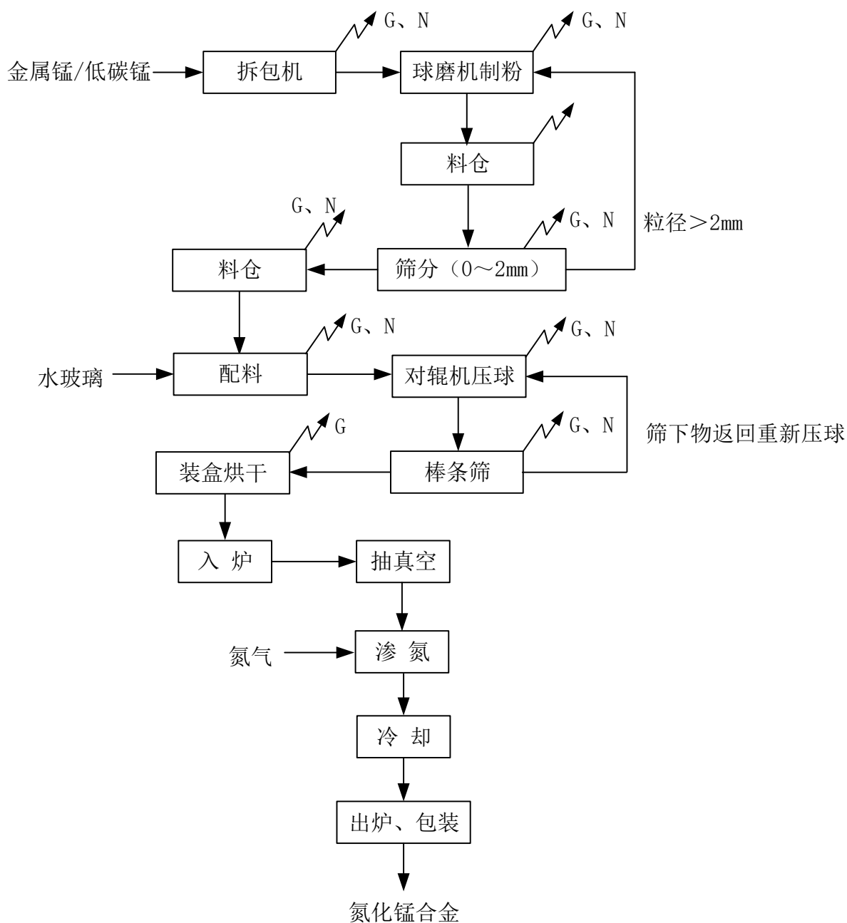
图 3.3-1 本项目生产工艺流程图及产排污环节
