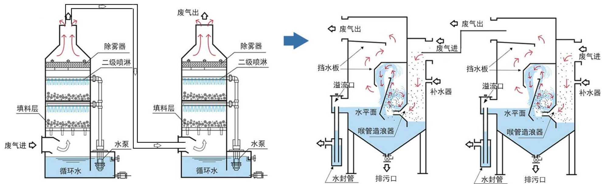
图 6.2-1 二级水浴除尘器工作原理图
