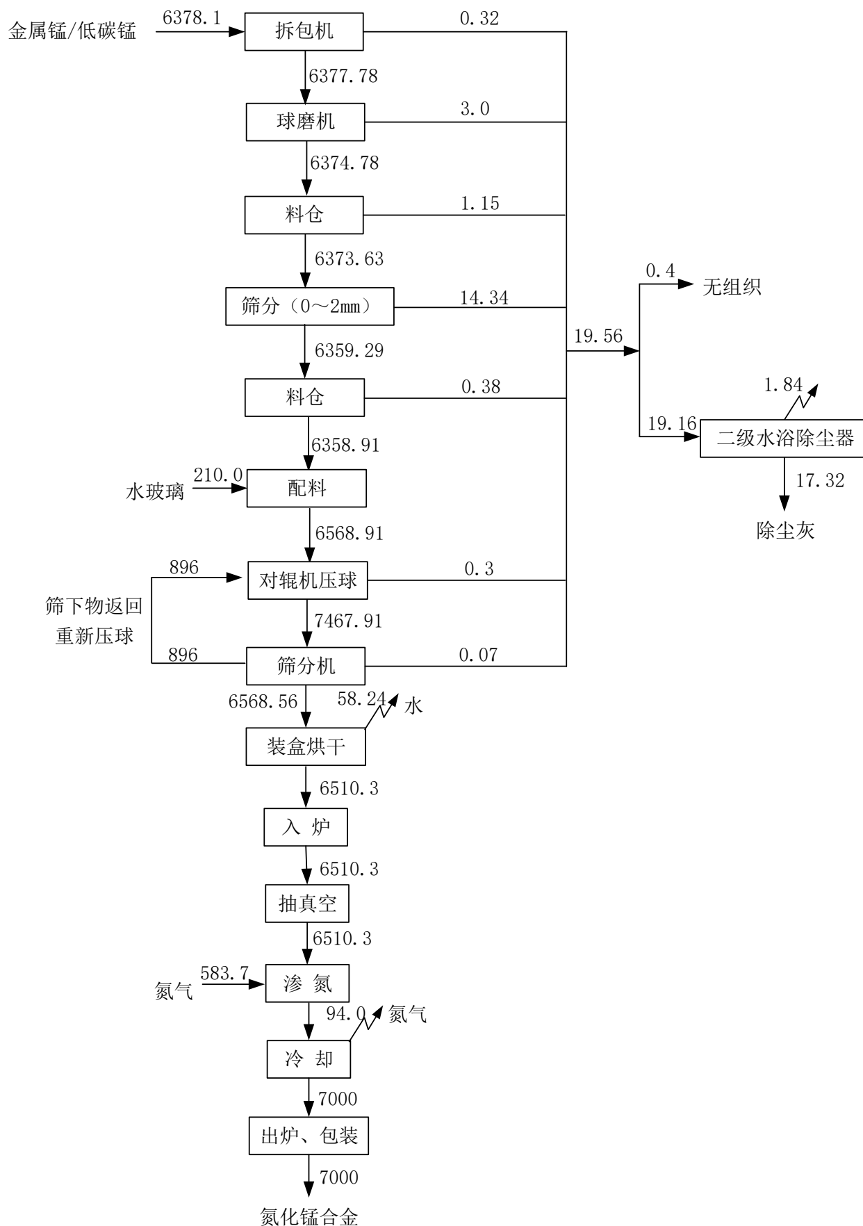
图 3.4-1 本项目物料平衡图（单位：t/a）
