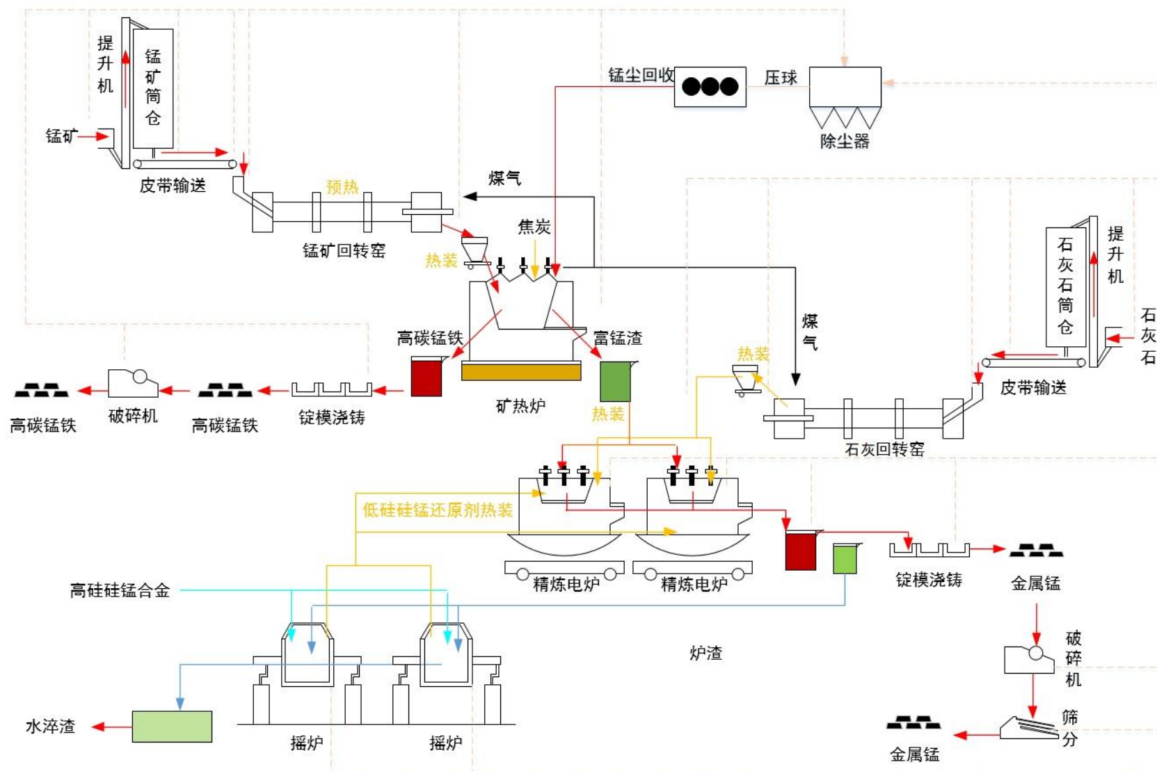
图 3.1-4 四车间一期生产工艺流程图
