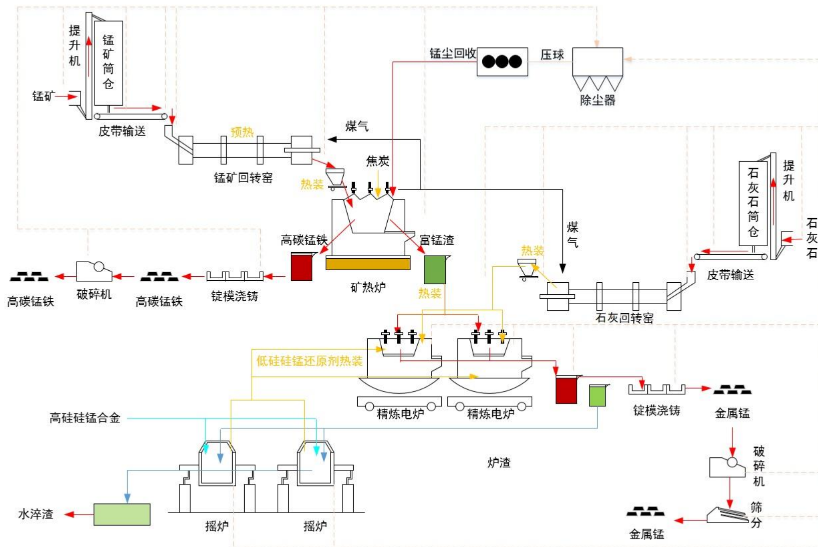
图 3.1-3 三车间生产工艺流程图
