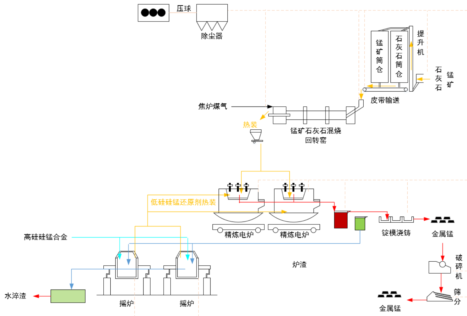
图 3.1-5 四车间二期生产工艺流程图
