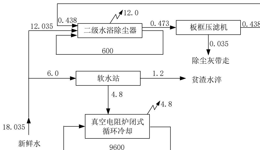
图 3.5-1 本项目水平衡图 (单位: t/d)
