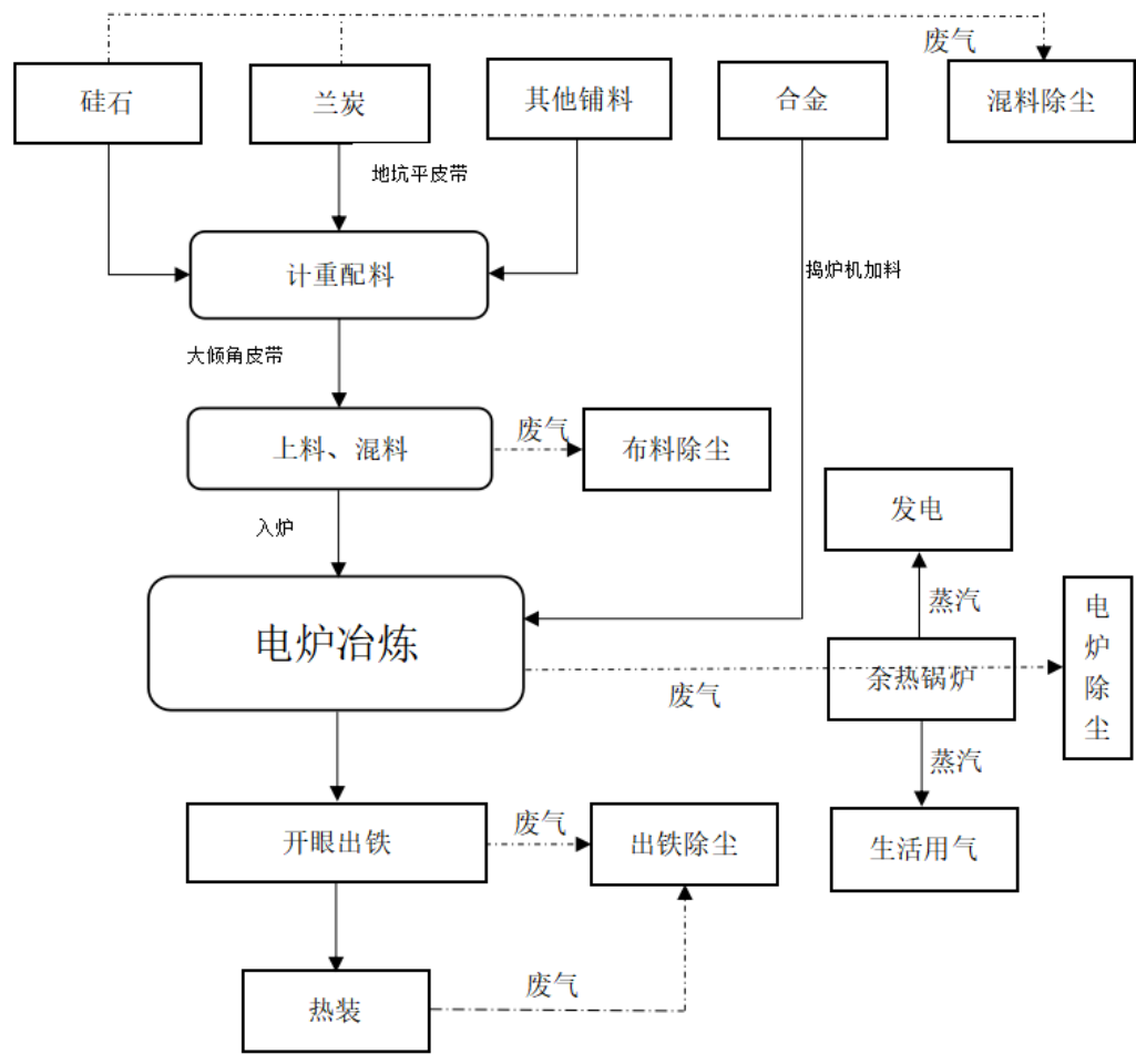
图 3.1-6 液态高硅硅锰合金生产工艺流程及产污环节示意图
