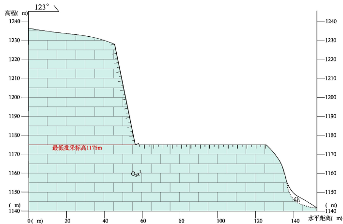
图 7-7 采场 1 地质剖面图
