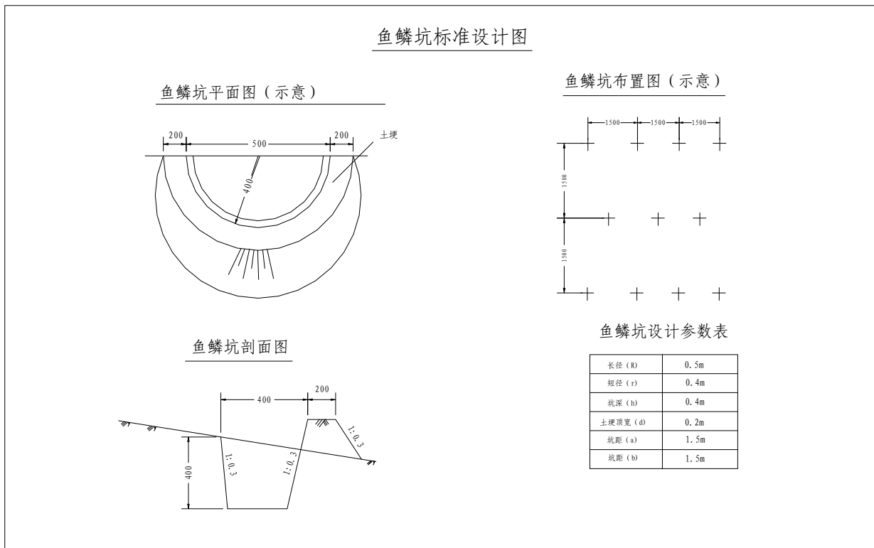
图 10-1 鱼鳞坑典型示意图
