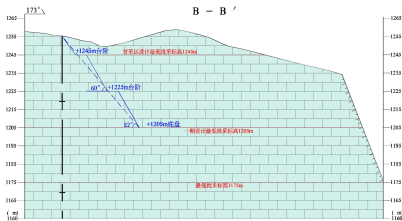
图 7-6 终了边坡地质剖面图
