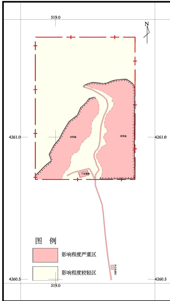
图 7-5 矿山地质环境影响程度现状评估综合分区图
