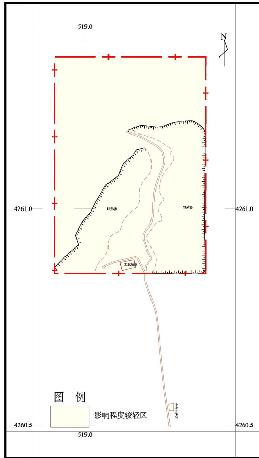
图 7-1 地质灾害现状评估分区图
