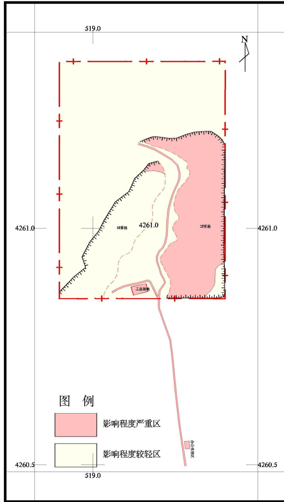
图 7-4 土地资源影响和破坏程度现状评估分区图
