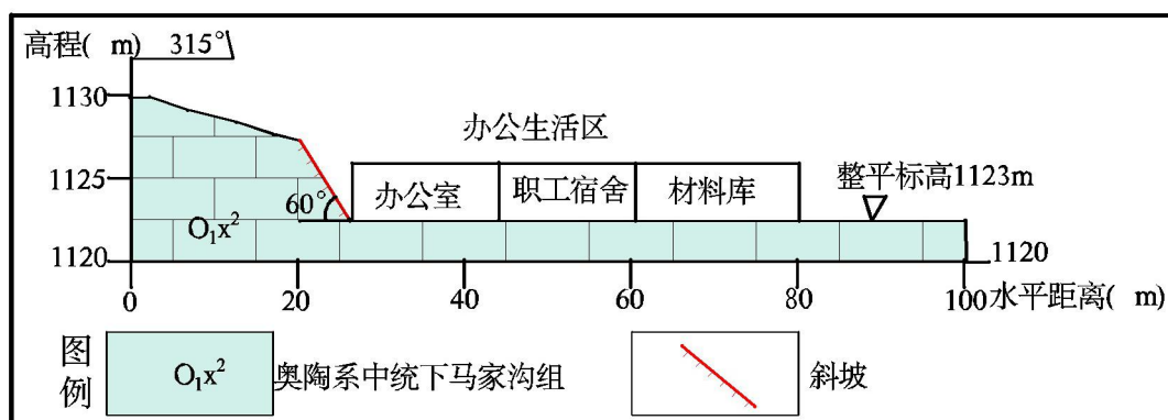
图 7-9 办公生活区地质剖面图
