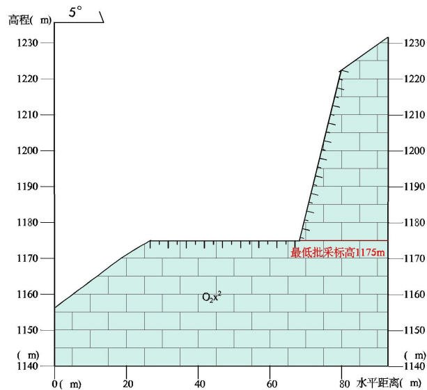
图 7-8 采场 2 地质剖面图
