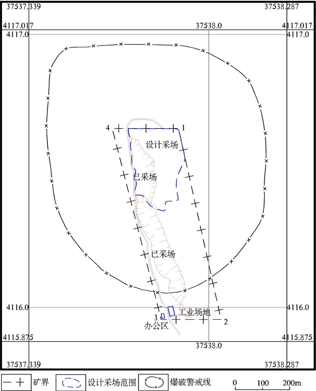
图 5-1-1 矿区爆破警戒线分布图
