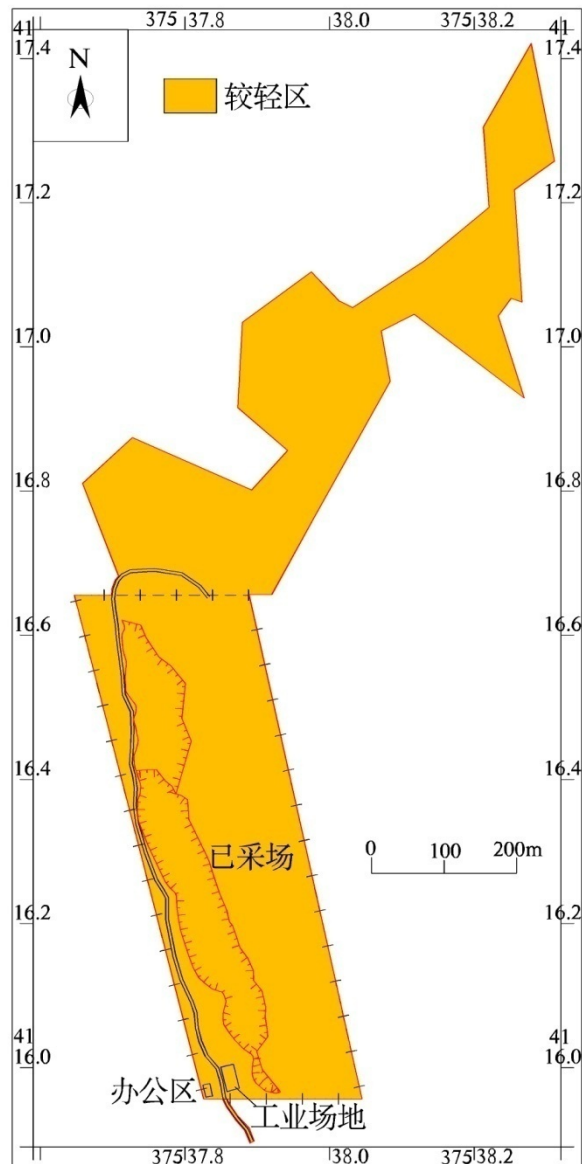
图 8-2-2 含水层现状评估图
