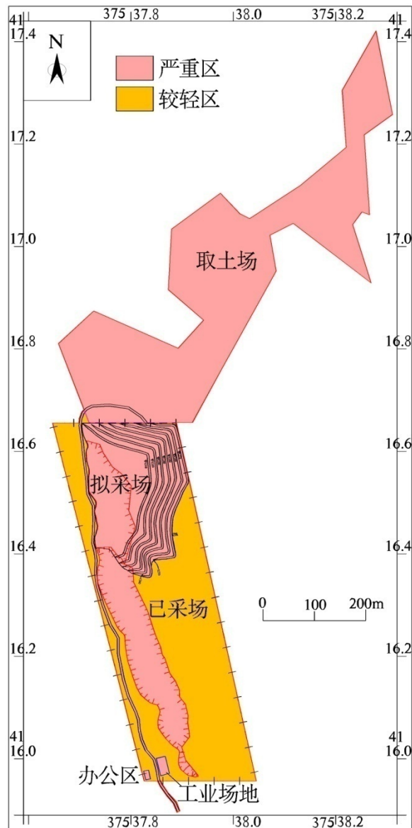
图 8-3-3 采矿活动对地形地貌景观预测评估分区图
