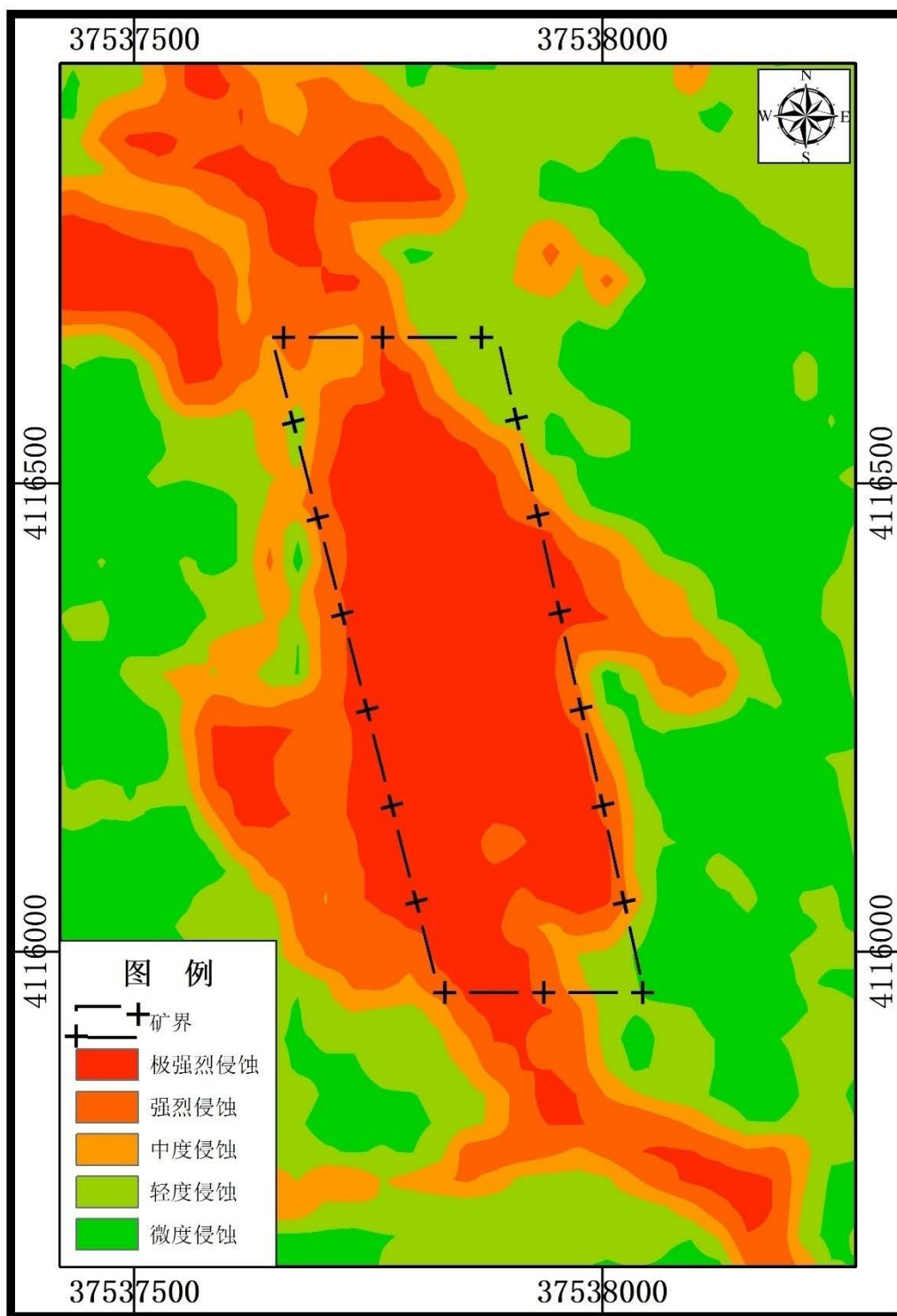
图 2-4-2 土壤侵蚀现状图
