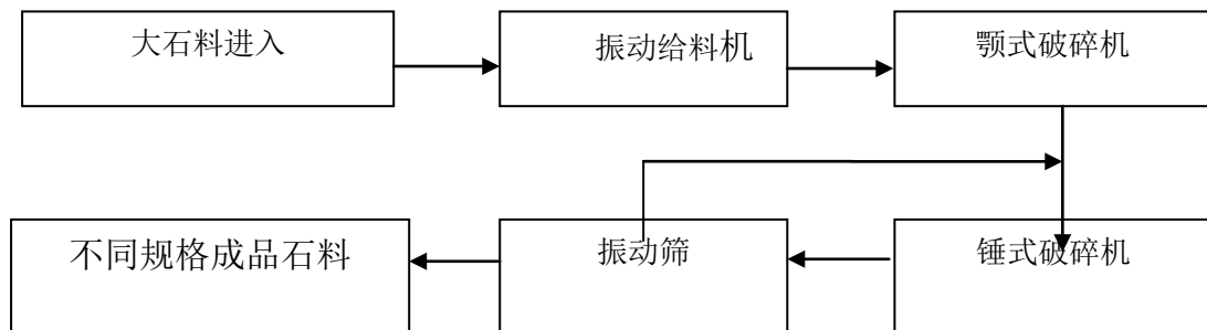
图 1-1-1 生产线流程图
