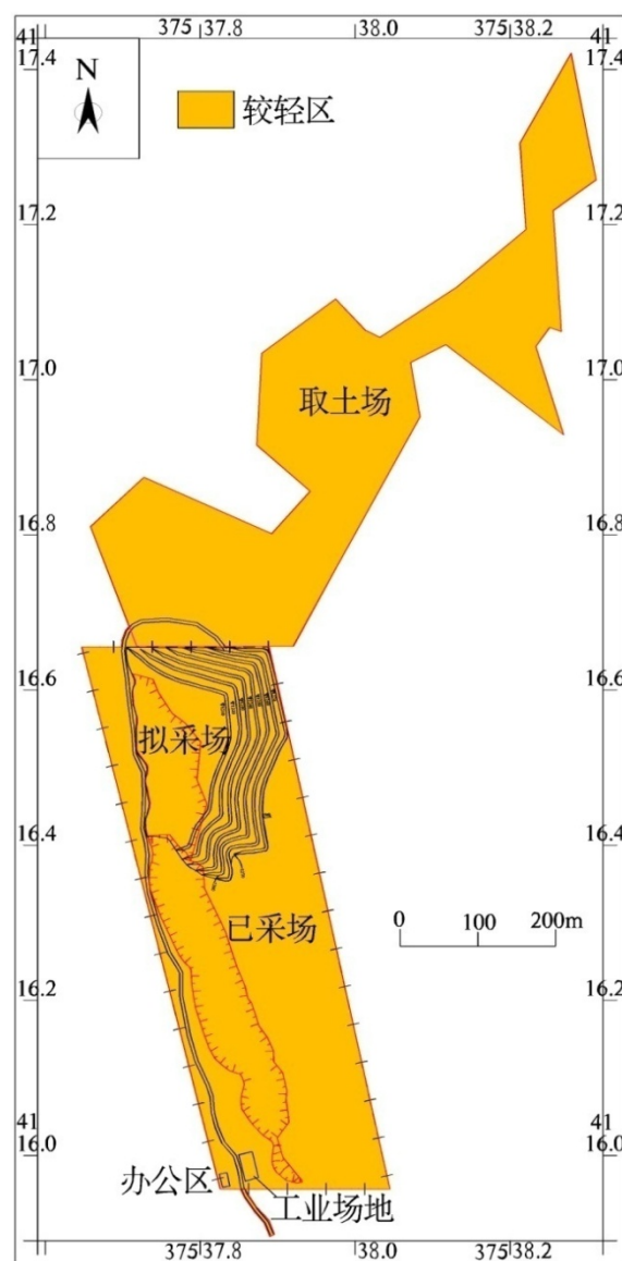
图 8-3-1 服务期评估区地质灾害危险性预测评估分区图
