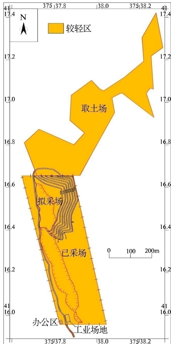
图 8-3-2 服务期内采矿活动对含水层影响分区图
