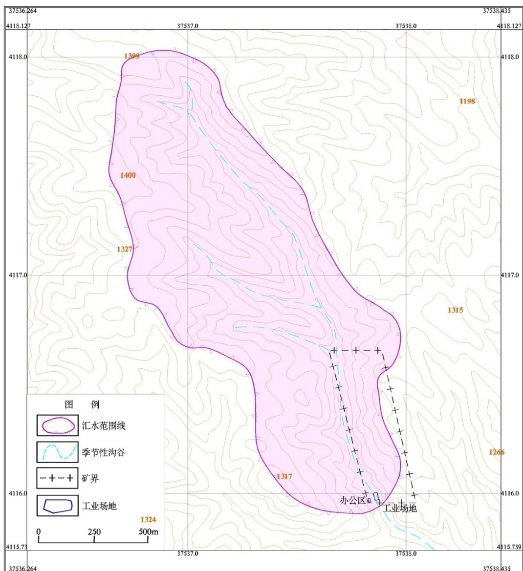
图 8-3-1 工业场地所在沟谷汇水范围图
